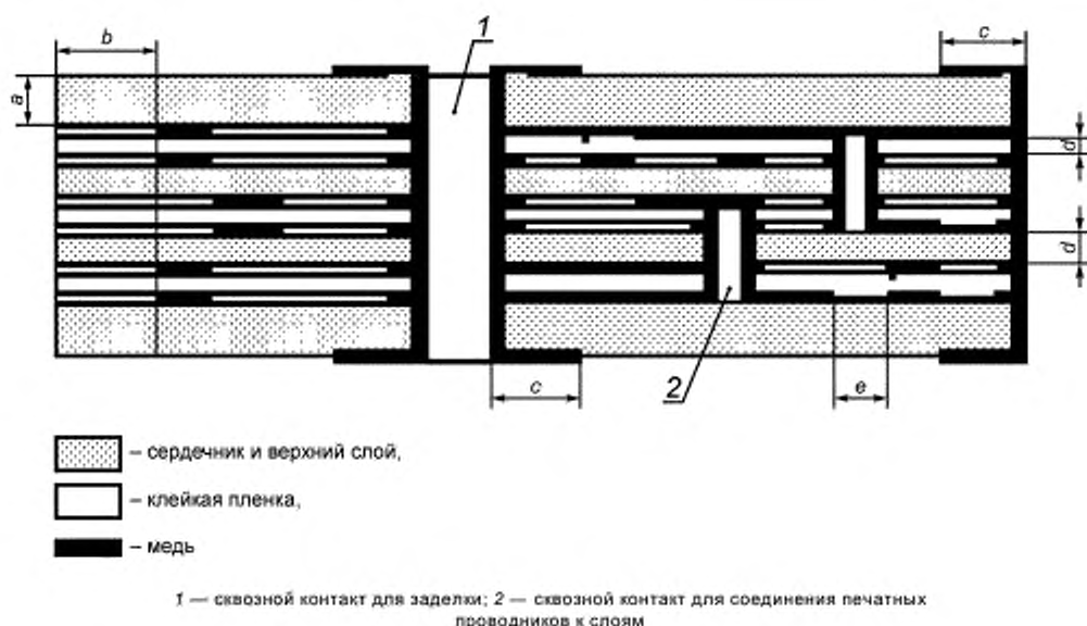
Рисунок 4 — Минимальные расстояния для многослойных печатных монтажных плат
