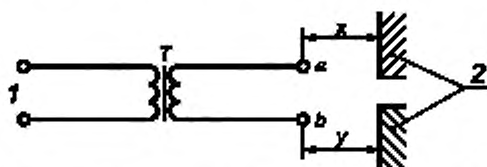
Рисунок 10 — Схема для испытания выключателей питания
