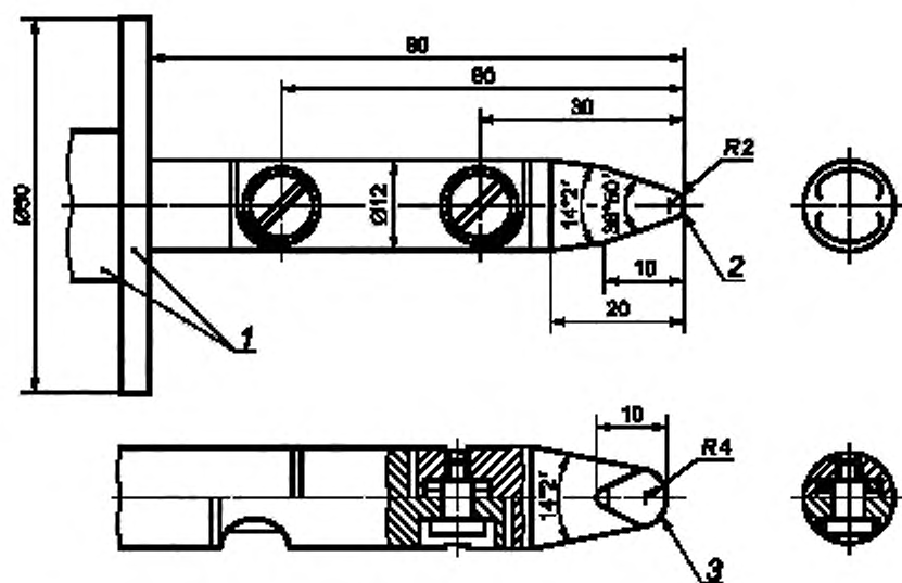
1 — изоляционный материал. 2 — цилиндрическая форма; 3 — сферическая форма
