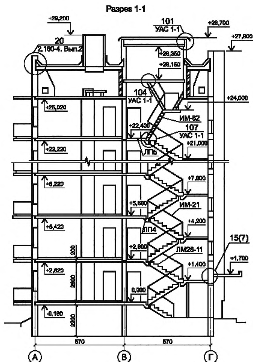
Рисунок Г.3 — Пример выполнения разреза жилого дома
