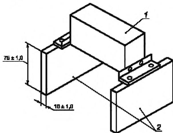
Рисунок 2 — Устройство для тепловых испытаний
