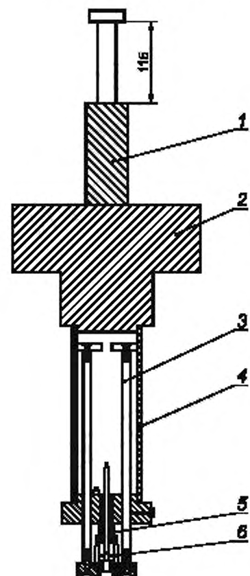
1 — падающий груз (1 кг); 2 — статический груз (9 кг); 3 — шток скольжения; 4 — обойма; 5 — уплотняющая головка (подогнана к диаметру тигля с зазором 0,5 мм); 6 — тигль с загрузкой и мешалкой
