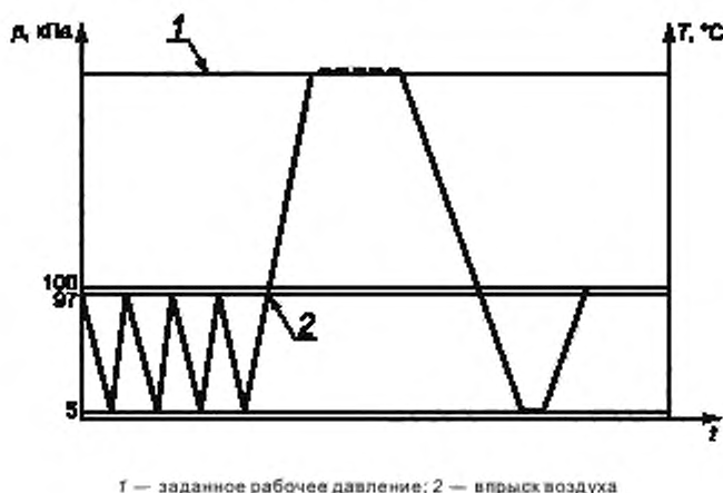
Рисунок В.1 — Стандартный испытательный цикл — удаление воздуха при доатмосферном давлении
