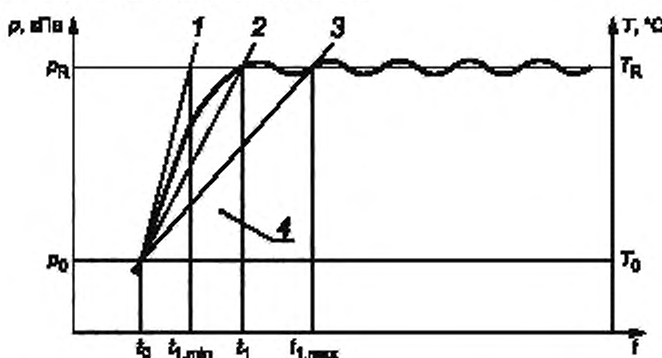
1 — максимальная скорость подъема давления на стадии подачи пара (p_R - p_0)/(t_{1,\min} - t_0) ; 2 — усредненная скорость подъема давления; 3 — минимальная скорость подъема давления на стадии подачи пара (p_R - p_0)/(t_{1,\max} - t_0) ; 4 — интегральная выдержка на стадии подъема температуры ICE (Integrated come — up Exposure): площадь между T_0 и кривой T_C на участке от точки t_0 до точки t_1 ; p_R — давление насыщенного пара, соответствующее заданной рабочей температуре (заданное рабочее давление в камере), кПа; p_0 — давление насыщенного пара, соответствующее температуре T_C = T_0 , кПа
