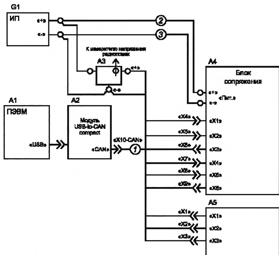
A1 — ПЭВМ; A2 — модуль USB-to-CAN; A3 — V-образный эквивалент сети по ГОСТ Р 51319; A4 — блок сопряжения; A5 — испытуемая АС; G1 — источник питания; 1 — кабель; 2, 3 — провод ML-4G
