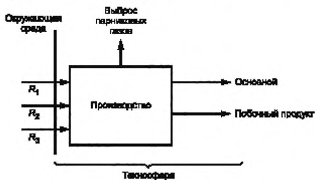
Рисунок 2 — Многовыходная система
