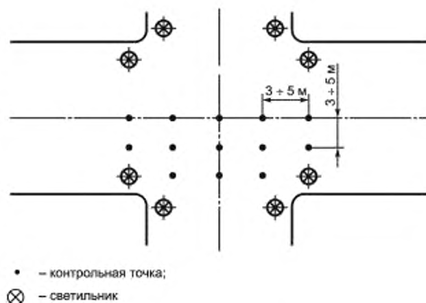
Рисунок А.6 — Расположение контрольных точек при измерении средней освещенности улиц на перекрестке
