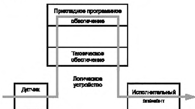
Рисунок С.1 — Логическое решающее устройство
