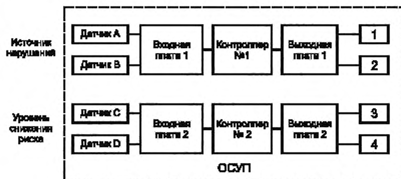
Рисунок 2 — Функция ОСУП и независимость источника нарушений
