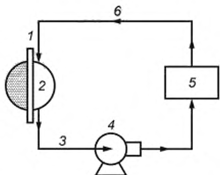
1 — подача среды-носителя на повторный цикл; 2 — камера с изнаночной стороны элементарной пробы для взятия пробы среды-носителя; 3 — взятие пробы среды-носителя; 4 — насос; 5 — анализатор проб среды-носителя (неразрушающий); 6 — среда-носитель после анализа
