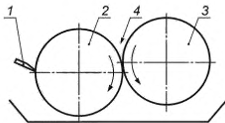
1 — рапель, 2 — дукторный валик, 3 — наносный валик, 4 — зона затягивания
