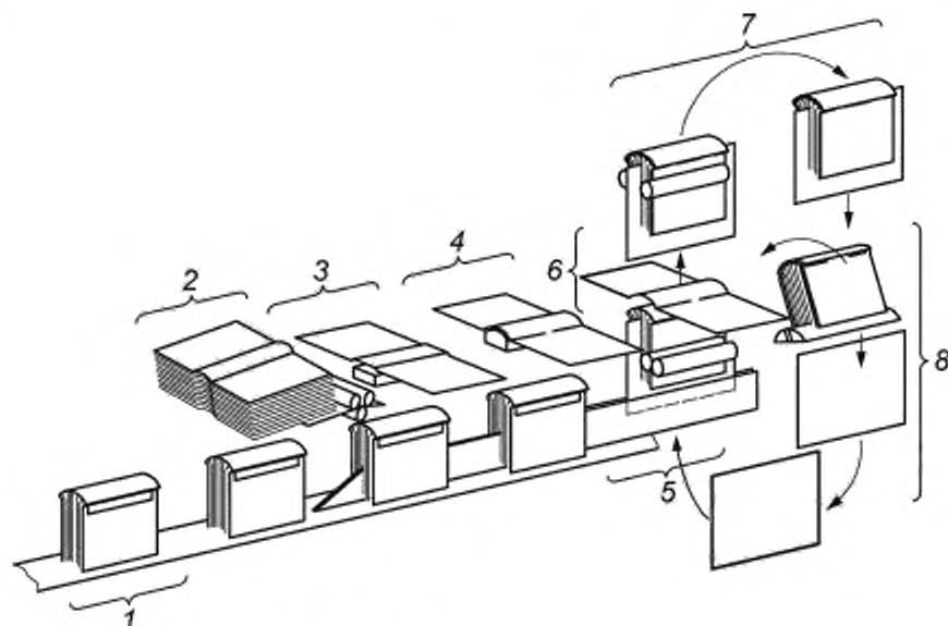
1 — ввод блока; 2 — самонаклад переплетных крышек (и каландрирование); 3 — секция биговки переплетных крышек; 4 — секция кругления корешка переплетных крышек; 5 — секция промазки клеем; 6 — секция вставки блока в переплетную крышку; 7 — секция обжимки (обкатки); 8 — вывод
