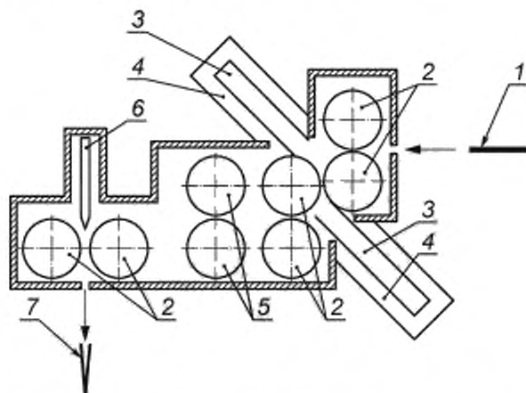
1 — несфальцованный лист; 2 — фальцевальные валики; 3 — фальцкассета; 4 — звукозащитный кожух; 5 — резальное, перфорирующее, бигвальное устройство; 6 — фальцнож; 7 — сфальцованный лист
