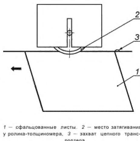
Рисунок 8 — Ролик для контроля толщины скomплектованного изделия
