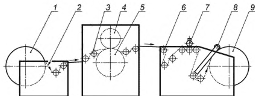
1 — устройство размотки рулонов; 2 — бумажная лента; 3 — валик для регулирования натяжения, 4 — тиснильный вал; 5 — опорный вал, 6 — направляющие валики, 7 — узел резки; 8 — приводной тянущий валик; 9 — устройство намотки рулонов
