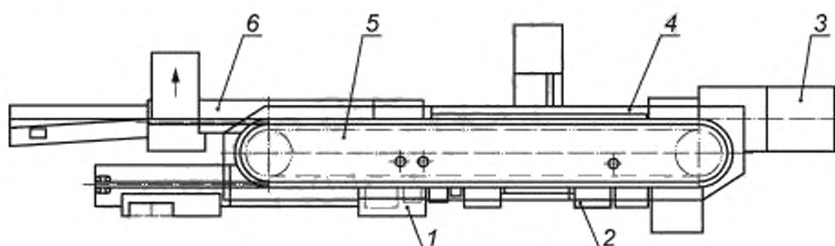
1 — секция фрезерования; 2 — клеевая секция; 3 — самонаклад обложки; 4 — обжимная секция; 5 — зажимы книжного блока; 6 — приемно-выводное устройство
