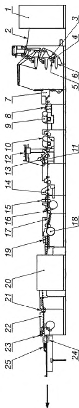
1 — установка для размотки рулонов; 2 — бумажная лента; 3 — опорный (печатный) цилиндр; 4 — формный цилиндр; 5 — аксиальный (распределитель) вал; 6 — печатная секция; 7 — поперечная беговая; 8 — продольная высека; 9 — секция фасонной высека; 10 — секция высека окошек; 11 — секция подачи материала окошек; 12 — размотка материала окошек; 13 — раковый аппарат; 14 — секция разводящая рубки; 15 — сегментный вал; 16 — секция загибки нижнего клапана; 17 — резиновые транспортирующие валы; 18 — каскадное колесо; 19 — валковый клеевой аппарат; 20 — устройство для сушки горячим воздухом; 21 — разделяющий вал; 22 — устройство для выравнивания; 23 — секция загибки закрывающего клапана; 24 — каскадный дисковый выклад; 25 — конвейер
