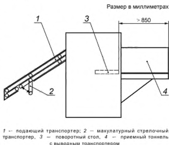
Рисунок 29 — Приемно-комплектующее устройство
