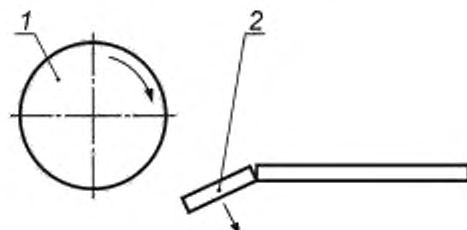
1 -- каскадный диск; 2 -- откидывающаяся крышка приемного стола
