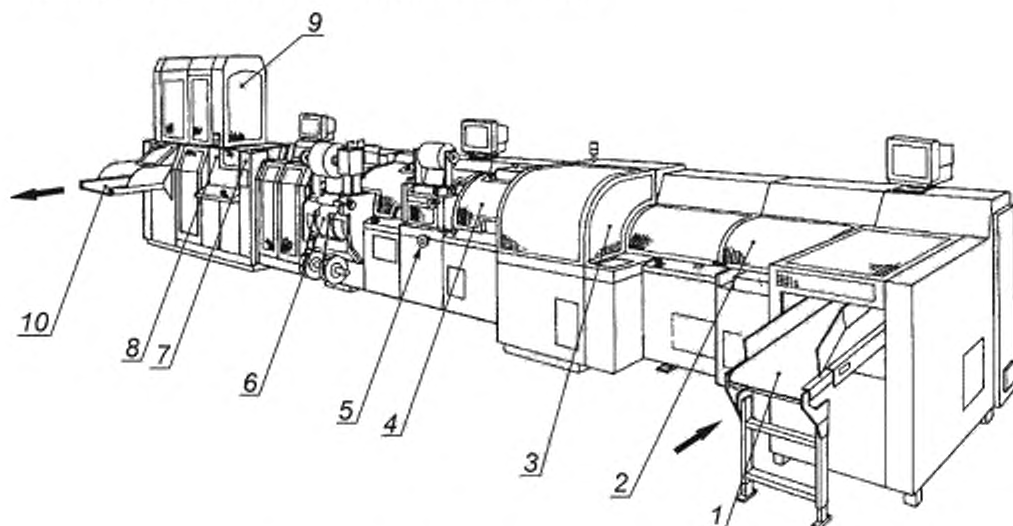
1 — загрузочный транспортер; 2 — нагреватель; 3 — секция кругления и обжимки; 4 — клеевая секция; 5 — марлевая секция; 6 — оклеивающе-капальная секция; 7 — магазин переплетных крышек; 8 — секция биговки, кругления переплетной крышки; 9 — секция вставки блока в переплетную крышку; 10 — выводной транспортер
