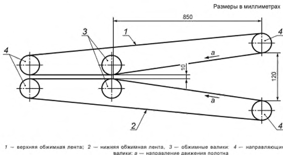
Рисунок 37 — Обжимной ленточный транспортер
