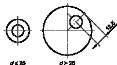
Рисунок 1 — Место вырезки образцов для сортового проката
