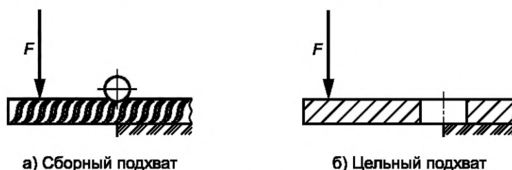
Рисунок 3 — Схема нагружения выпуска подхвата
