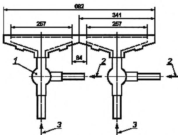
b — комбинация двух горелок, используемая при широкой ленточке
