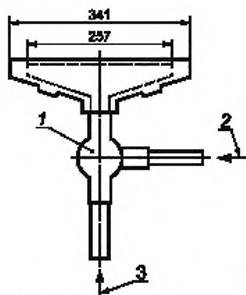
a — одиночная горелка, используемая при стандартной ленточке
