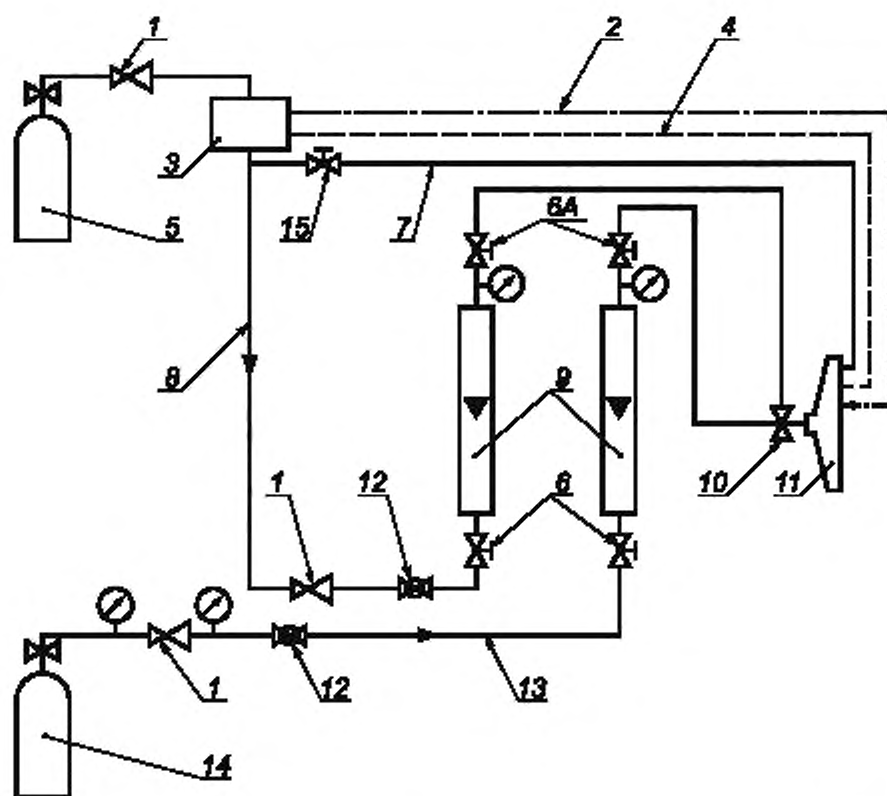
1 — регулятор; 2 — пьезоэлектрический воспламенитель; 3 — устройство для прерывания работы горелки; 4 — контрольные термодатчики; 5 — баллон с пропаном; 6 — винтовой клапан (6A — альтернативное расположение); 7 — вспомогательное питание; 8 — поступление газа; 9 — расходомер; 10 — смеситель Вентури; 11 — горелка; 12 — шаровой клапан; 13 — поступление воздуха; 14 — баллон со сжатым воздухом; 15 — винтовой клапан вспомогательного питания
