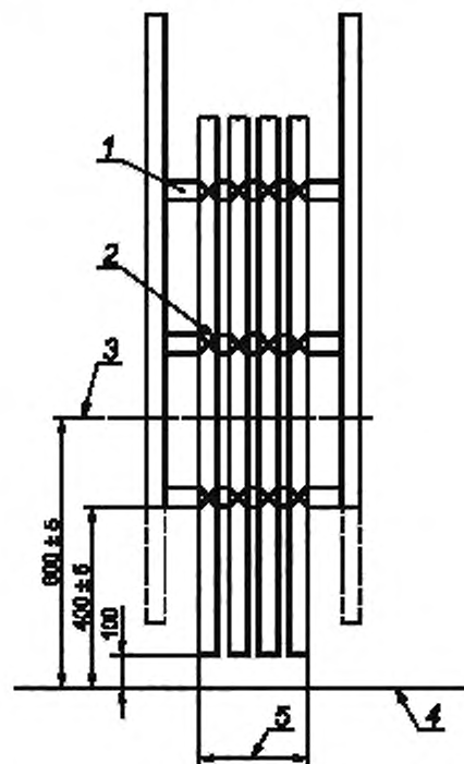
Рисунок 2 — Термоизоляция задней и боковых стенок испытательной камеры
