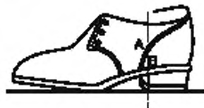
Рисунок 8 — Измерение перекаса накладных задников (задников)
