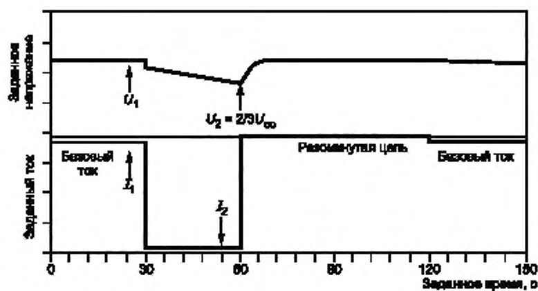
Рисунок 1 — Профиль испытания на пиковую мощность
