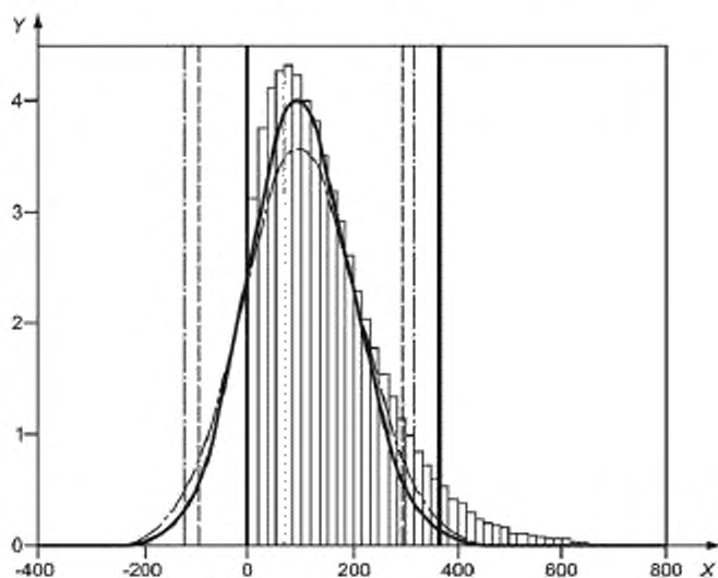
Рисунок 13 — То же, что и на рисунке 11, но для x_1 = 0,010 и с двумя кривыми, полученными способом оценивания по GUM (высокий пик — учтены только члены 1-го порядка; низкий пик — учтены члены более высокого порядка)
