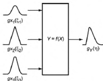
Рисунок 2 — Трансформирование распределений трех ( N = 3 ) независимых входных величин
