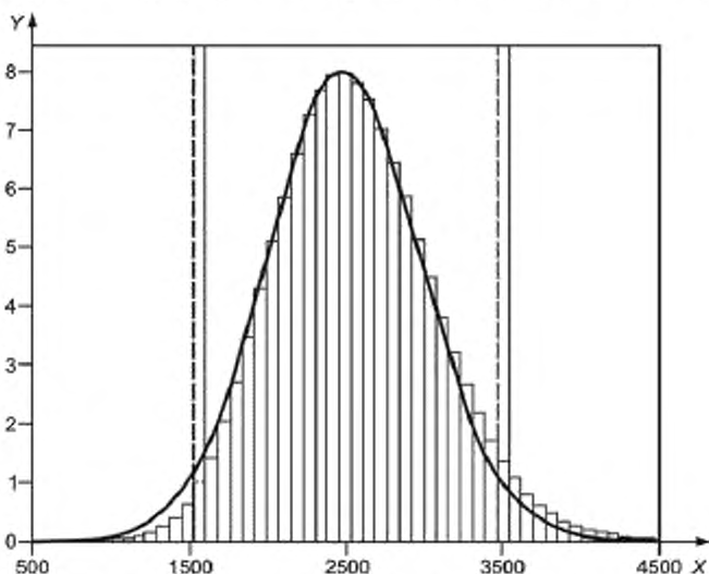
Рисунок 14 — То же, что и на рисунке 13, но для x_1 = 0,050
