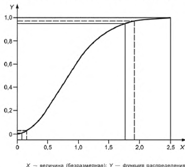
Рисунок 1 — Функция распределения G_Y(\eta) , вероятностно симметричный и наименьший 95 %-ные интервалы охвата
