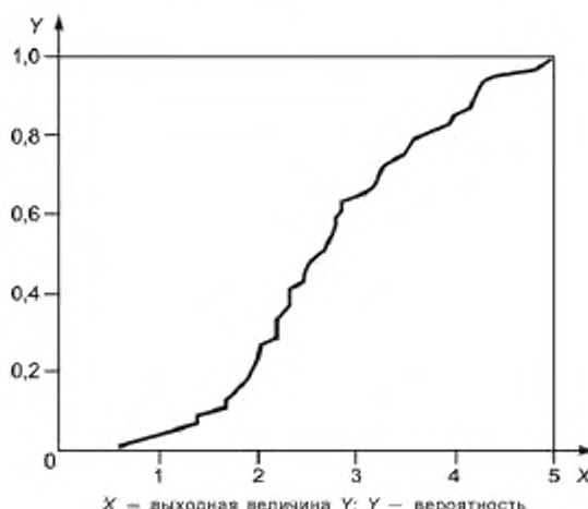
Рисунок D.1 — Аппроксимация \tilde{G}_Y(\eta) функции распределения G_Y(\eta)
