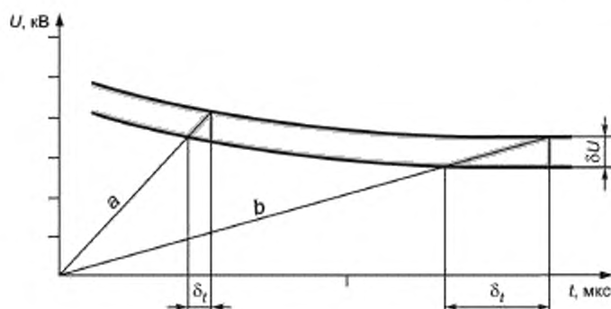
Рисунок 8 — Типичная кривая разрядника
