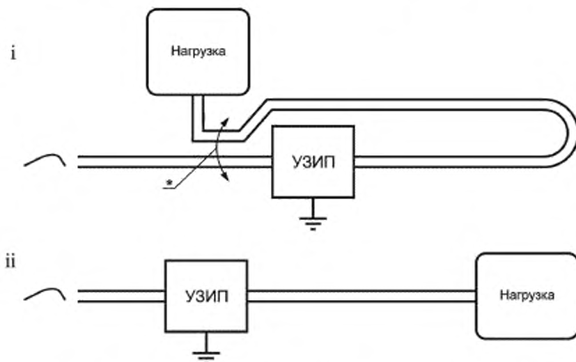
Рисунок К.7б — Примеры правильной и неправильной установок УЗИП с точки зрения индуктивной связи
