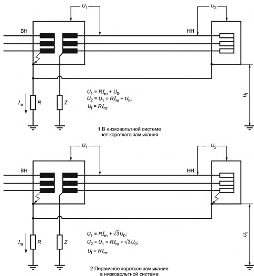
Рисунок Е.9 — Система IT, пример е1
