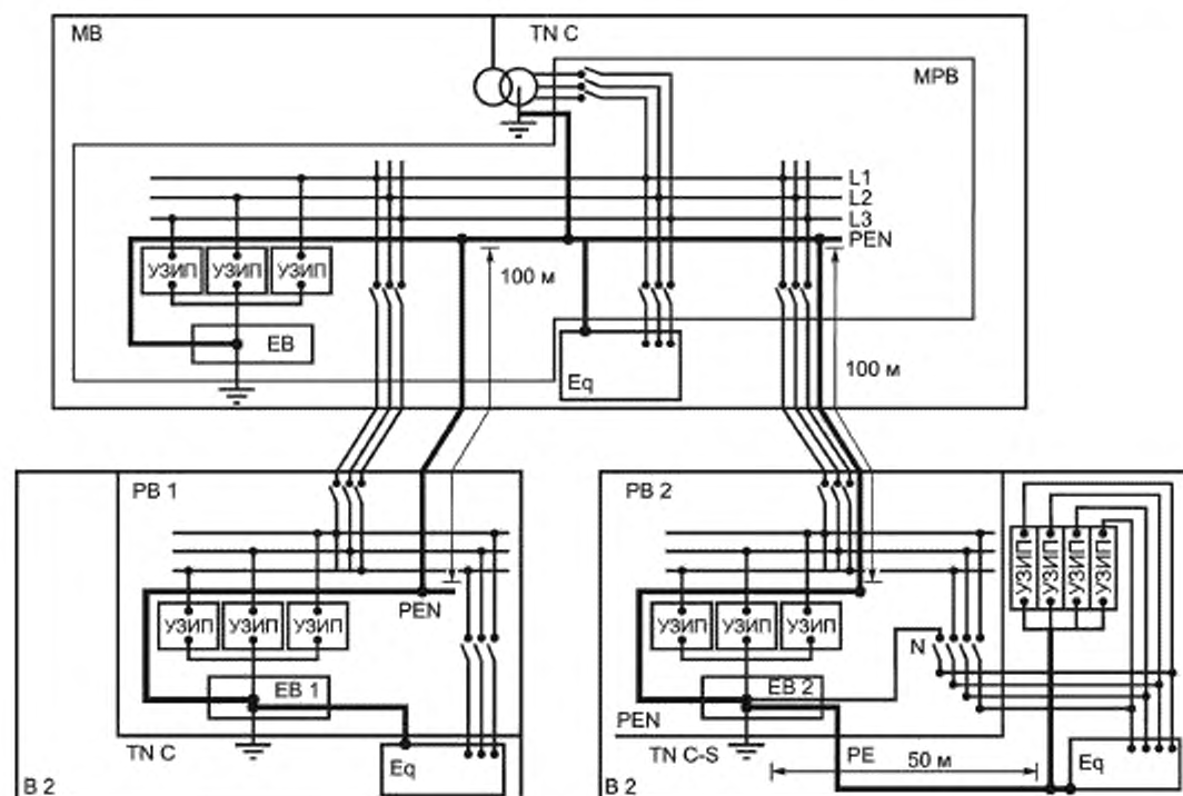
МВ — главное здание; В 1, В 2 — производственные здания; ЕВ, ЕВ 1, ЕВ 2 — эквипотенциальные соединительные шины; РВ 1, РВ 2 — распределительные щиты; Ек — электрооборудование и нагрузки; TN C, TN C-S — системы питания и заземления
