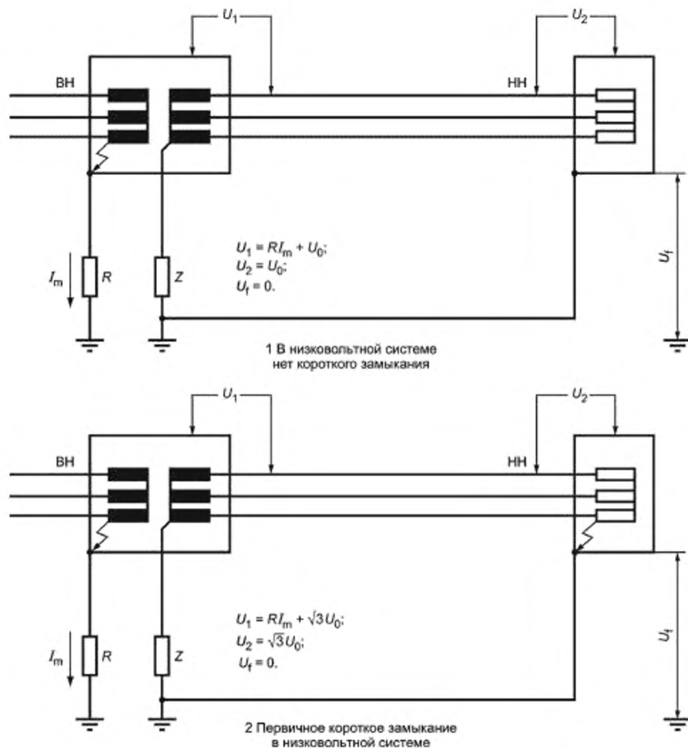
Рисунок Е.8 — Система IT, пример d
