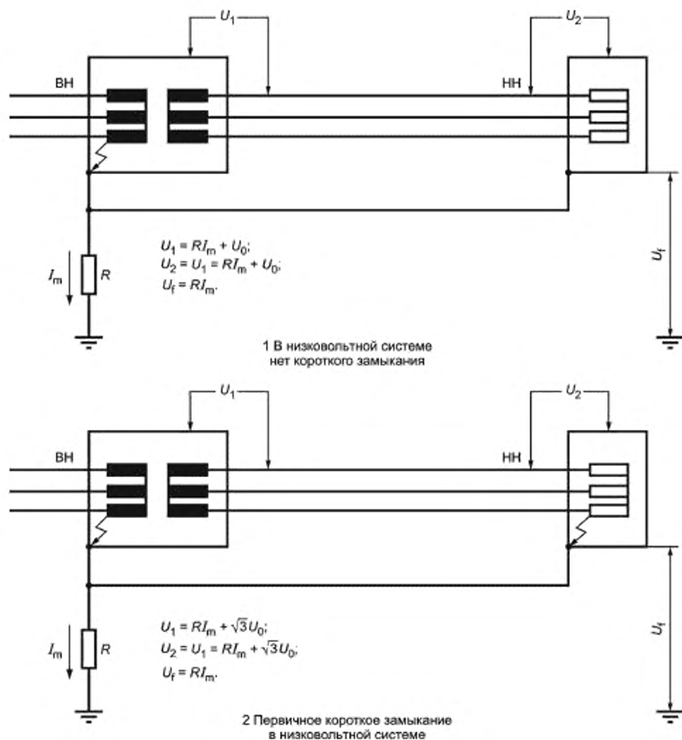
Рисунок Е.10 — Система IT, пример е2
