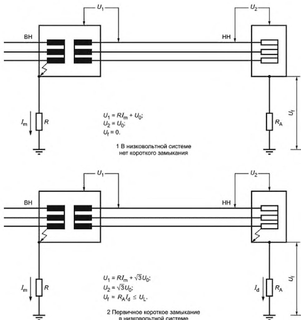
Рисунок Е.7 — Система IT, пример с2
