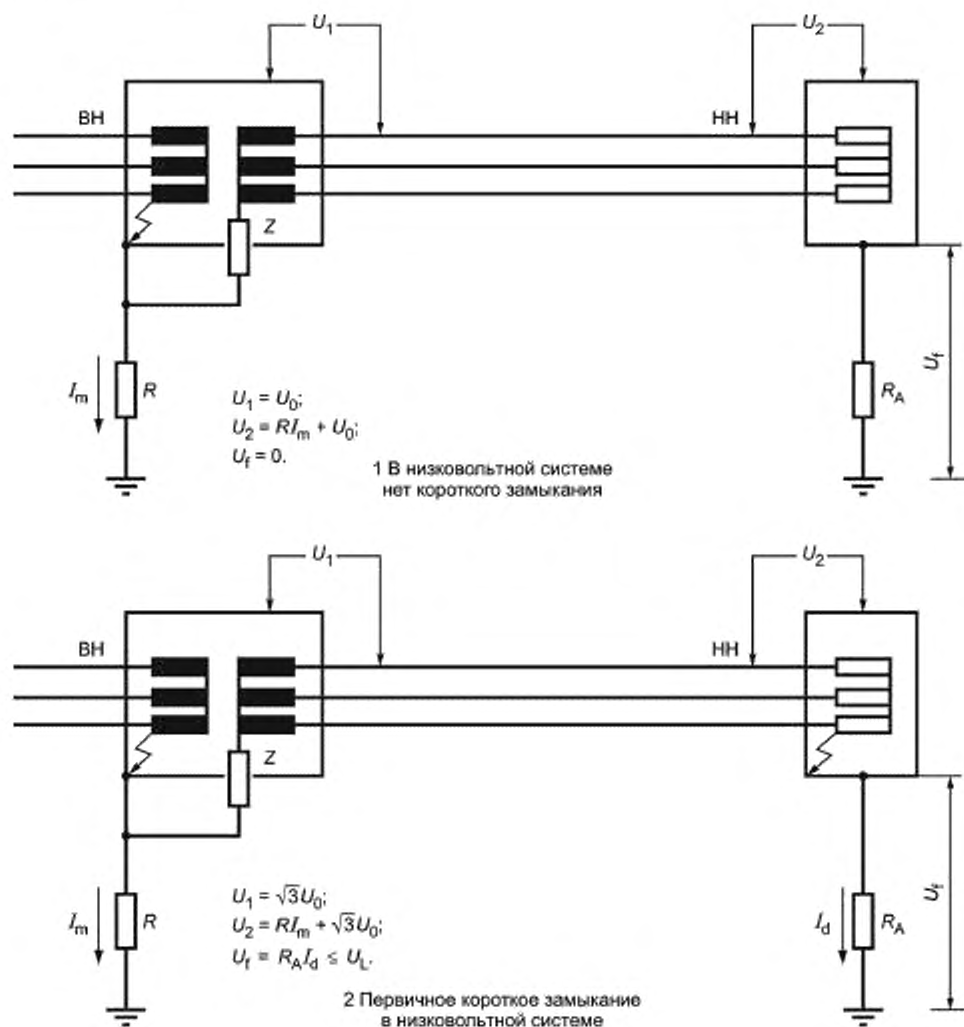
Рисунок Е.5 — Система ГТ, пример б
