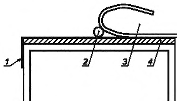
1 — нижняя простыня; 2 — сигарета, помещенная на стыке нижней простыни; 3 — постельные покрывала (сложенные вдвое); 4 — подложка для испытаний
