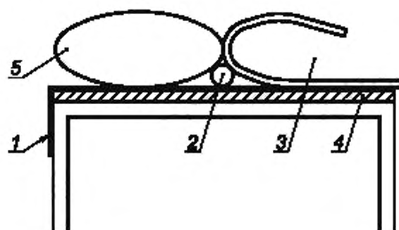
1 — нижняя простыня; 2 — сигарета, помещенная на стыке подушки и постельных покрывал, 3 — постельные покрывала (сложенные вдвое); 4 — подложка для испытаний; 5 — подушка
