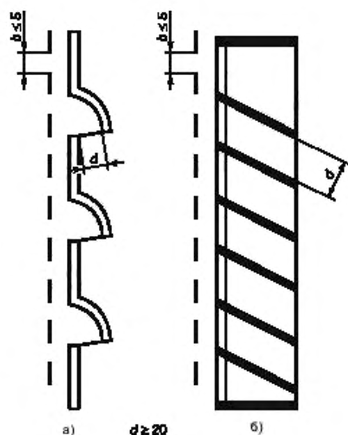
Рисунок А.16 — Вентиляционные отверстия для непищевой зоны
