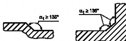
Рисунок А.3 — Пищевая зона. Сварное соединение с шлифованием и полированием сварного шва
