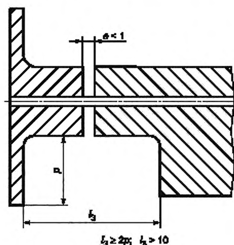
Рисунок А.17 — Шарнирное соединение
