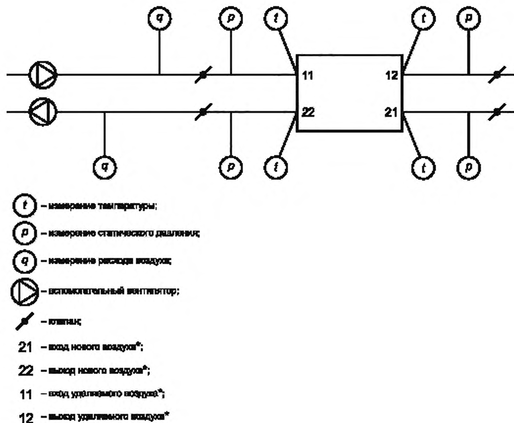
Рисунок 3 — Схема подключения оборудования и точки измерений
