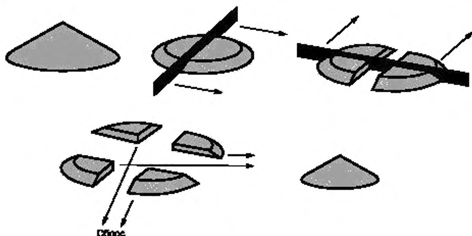
Рисунок 7 — Квартование
