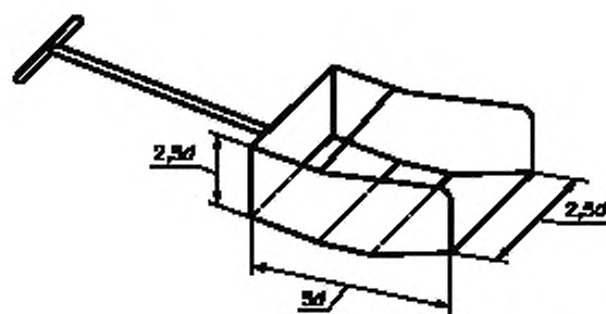
d — номинальный основной размер
