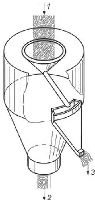
б) Тип с вращающимся потоком
