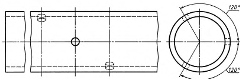
Рисунок Е.1 — Эталонный образец с тремя отверстиями
