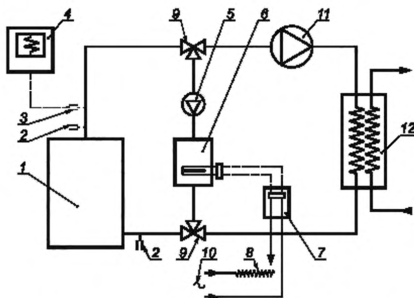
1 — испытуемый котел; 2 — датчики температуры; 3 — низкоинерционные термодатчики; 4 — самописец; 5 — насос; 6 — вспомогательный электрический котел; 7 — устройство для измерения электрической мощности; 8 — регулятор напряжения; 9 — клапаны с поворотом на 1/4; 10 — электропитание; 11 — дополнительный насос (при необходимости); 12 — система охлаждения (теплообменник)
