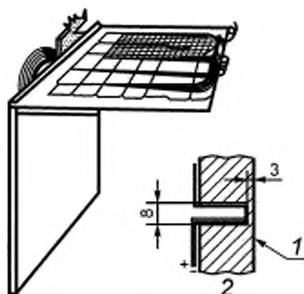
а) Компонировка установки с настенным монтажом приборов
