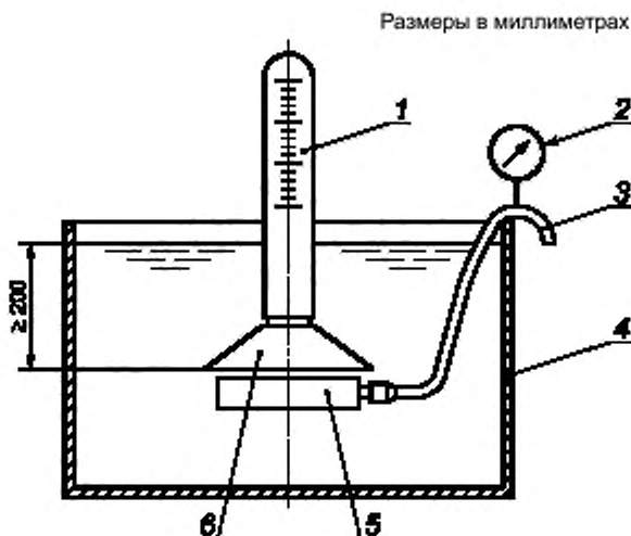
1 — градуированный баллон; 2 — калиброванный манометр; 3 — подача газа; 4 — резервуар с водой; 5 — редуктор (испытуемый образец); 6 — расструб
