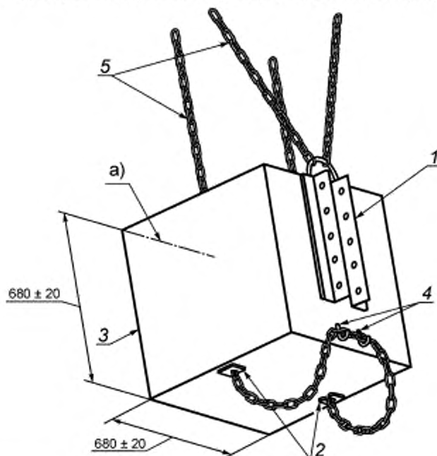
Рисунок 6 — Устройство подвеса блока маятника
