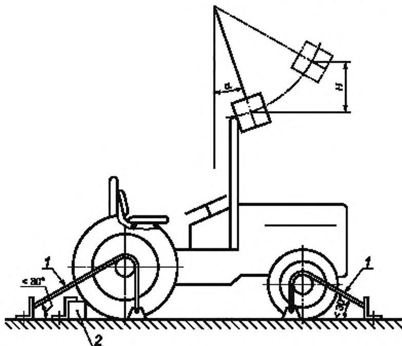
Рисунок 8 — Схема испытания защитного устройства при ударе спереди
