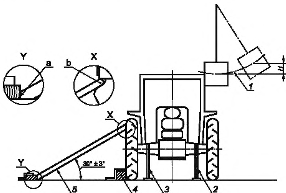
1 — дуга перемещения центра тяжести маятника при ударе, 2 — крепления трактора (см. 7.2.3); 3 — дополнительные крепления трактора, 4 — упорный брус; 5 — деревянный упор; а — заостренный торец упора, б — округленный торец упора для обеспечения контакта около края диска колеса
