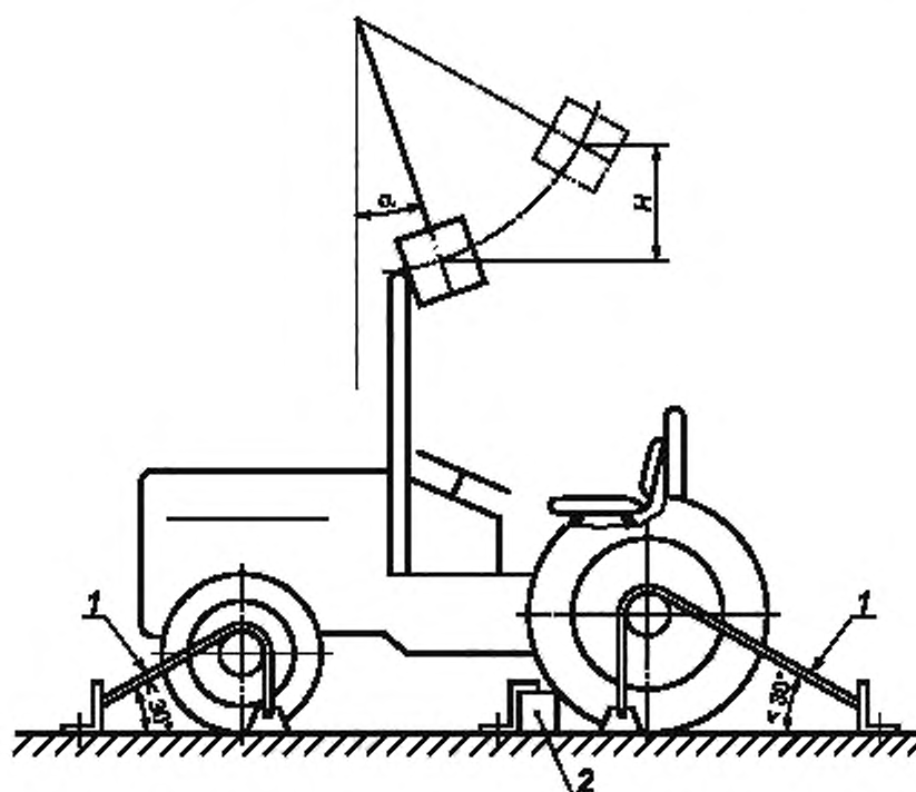
1 — крепления колес; 2 — упорный брус
