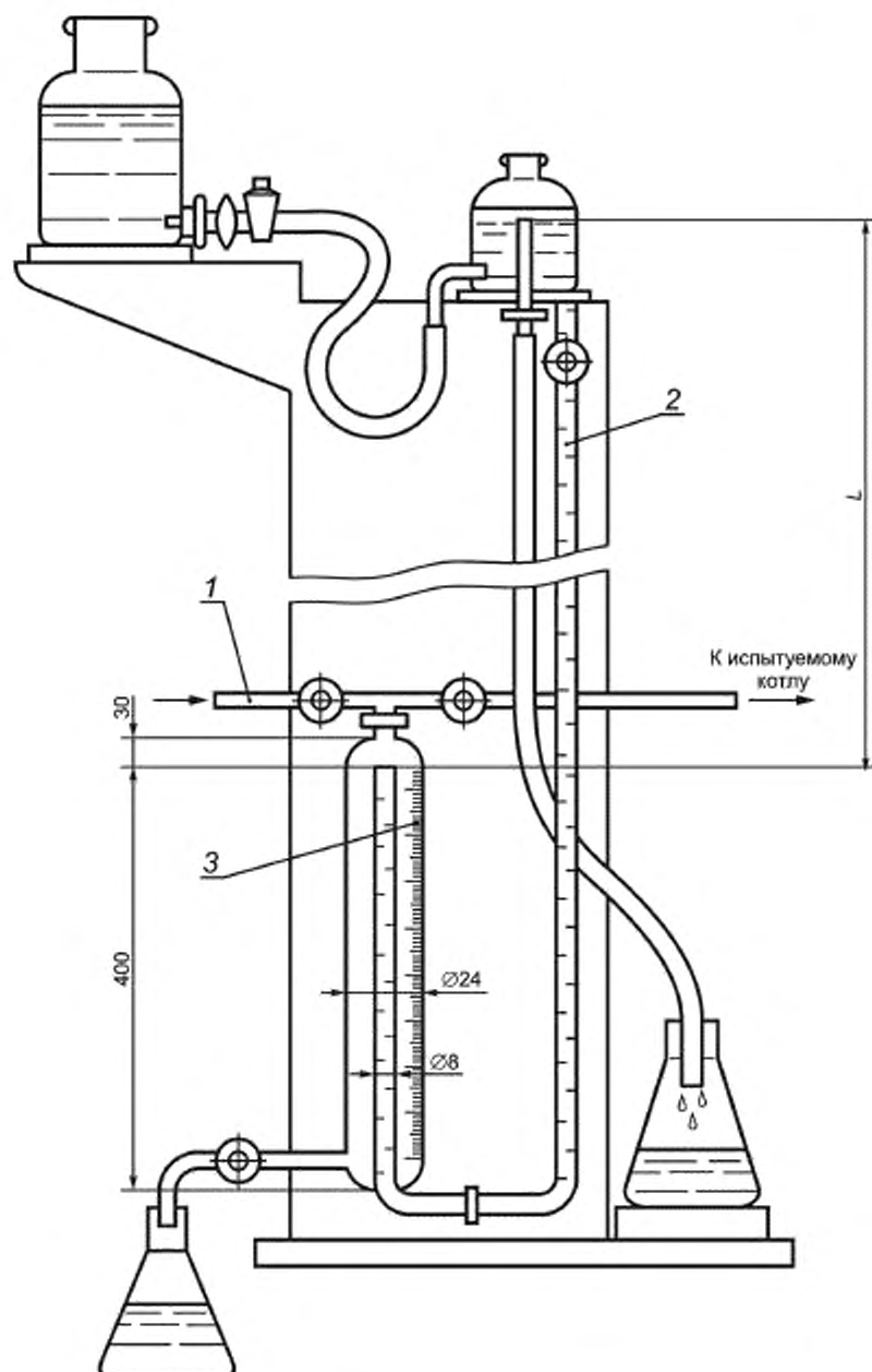
1 – сжатый воздух, 2 – градуированная шкала; 3 – измерительный сосуд
