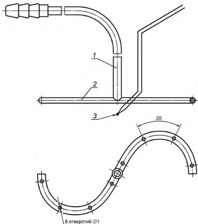
1 — медная трубка \varnothing 6 мм, 2 — медная трубка \varnothing 4 мм, 3 — термопара
