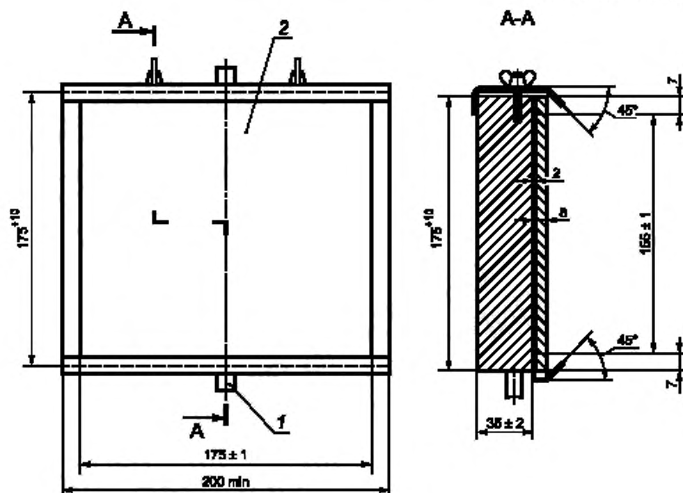
Рисунок 24 — Монтажная опора
