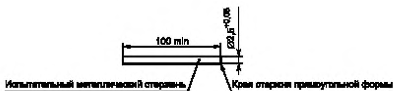
Рисунок 35 — калибр для проверки пазов, отверстий и обратных конусов
