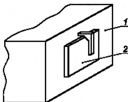
Рисунок 32 — Калибр для проверки габаритов крышек или закрывающих пластин
