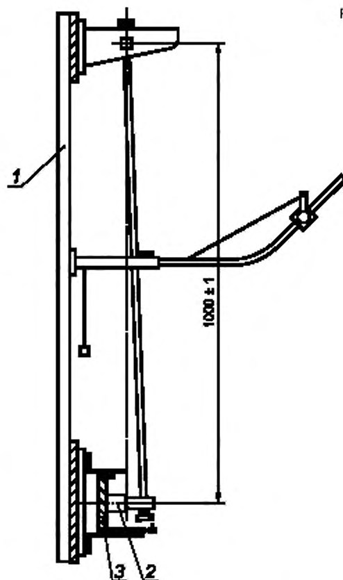
Рисунок 22 — Установка для проверки механической прочности соединителей
