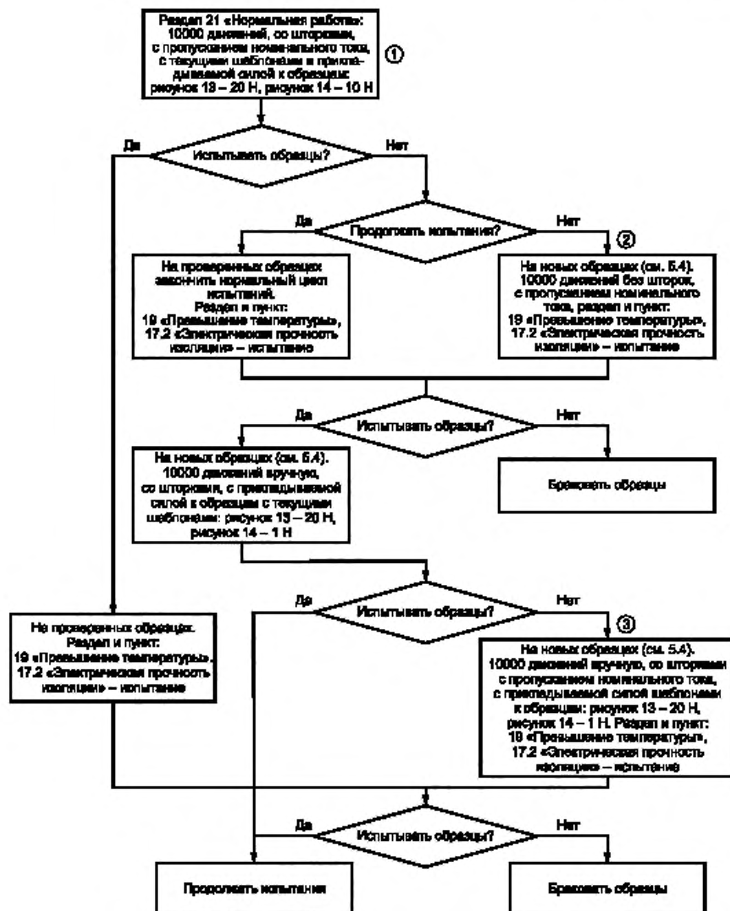
Рисунок 43 — Методика испытаний по разделу 21 «Нормальная работа»
