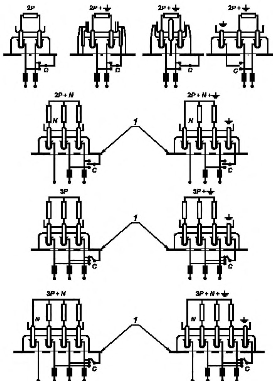
Рисунок 17 — Схема соединения для испытания соединителей на нормальную работу
