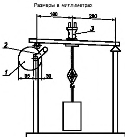
Рисунок 20 — Установка для испытания узла крепления шнура
