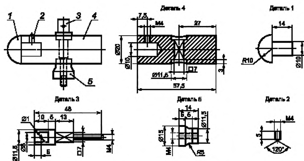
Рисунок 23 — Ударный элемент
