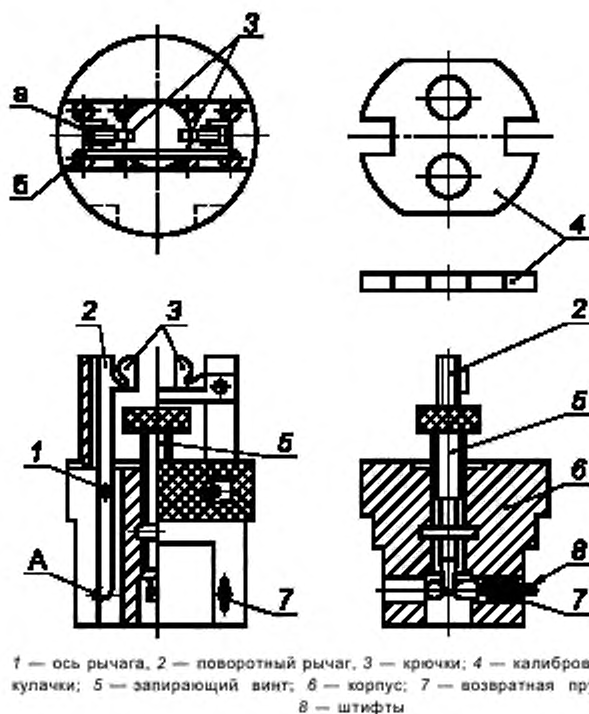
Рисунок ДА.10 — Установка для проверки усилия контактного нажатия боковых заземляющих контактов двухполюсных розеток на 10 и 16 А, 250 В
