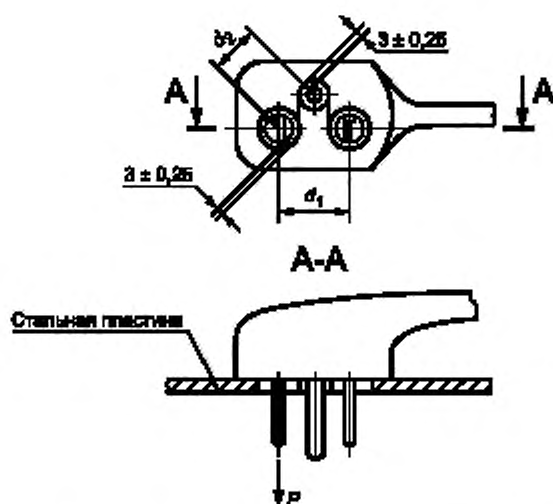
Рисунок 30 — Устройство для проверки механической прочности вилок
