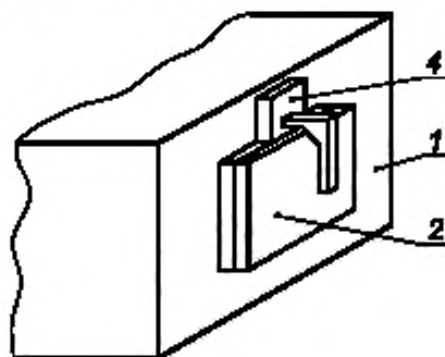
Рисунок 33 — Пример применения калибра на рисунке 32 к стационарным крышкам без винтов крепления к опорной или монтажной поверхности
