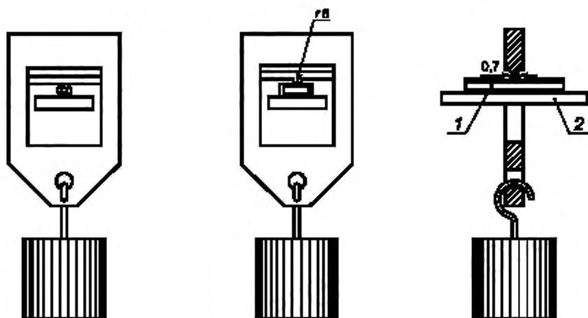
Рисунок 41 — Установка для испытания давлением при высокой температуре
