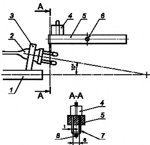
1 — основание; 2 — образец; 3 — зажим; 4 — груз; 5 — стержни; 6 — ось; 7 — стальная проволока; 8 — штырь вилки
