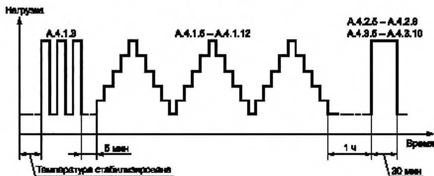
Рисунок A.1 — Рекомендованная последовательность испытаний для каждой температуры, когда все испытания выполняются в одном и том же устройстве
