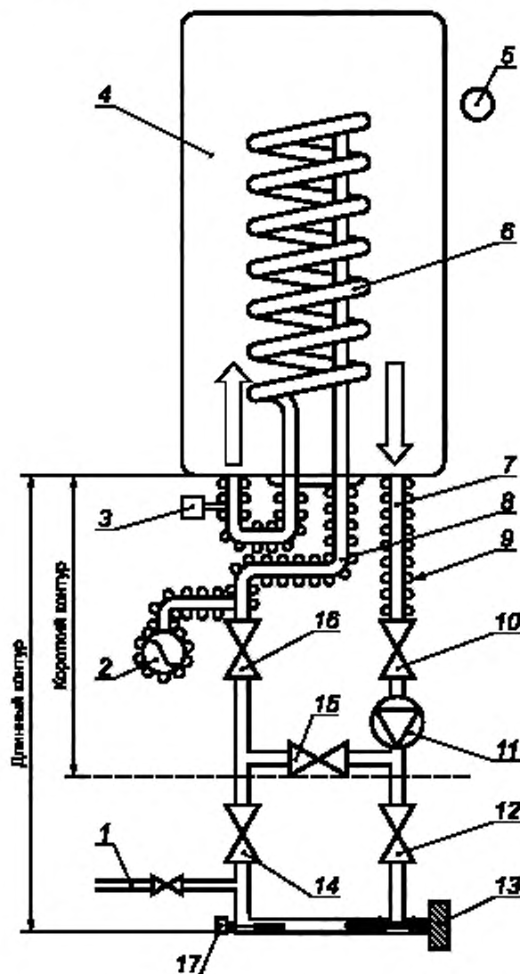
1 — подпиточная труба; 2 — изолированный расширительный бак; 3 — расширительный клапан; 4 — испытуемый резервуар; 5 — внешний термометр; 6 — нагревающий змеевик; 7 — точка измерения температуры T_g ; 8 — точка измерения температуры T_w ; 9 — теплоизоляция; 10, 12, 14, 15, 16 — клапаны; 11 — циркуляционный насос; 13 — электронагреватель; 17 — термостат
