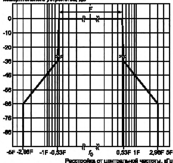
Рисунок 2 — Маска огибающей внеполосных радиосигналов в логарифмических координатах
