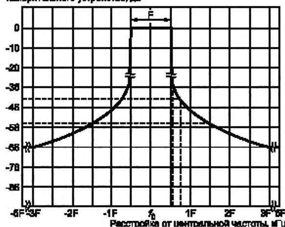
Рисунок 1 — Маска огибающей внеполосных радиоколебаний в линейных координатах
