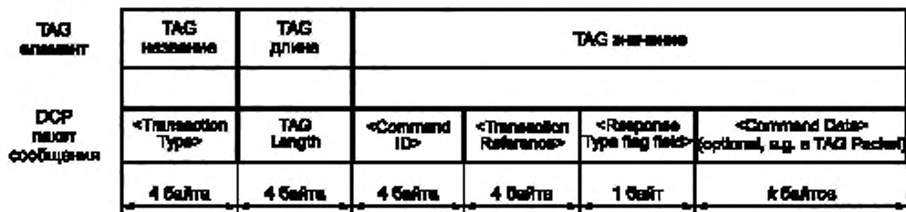
Рисунок Е.1 — Структура DCP пакета сообщения
