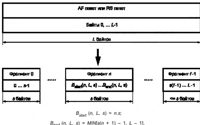
Рисунок 13 — Фрагментация AF или RS пакета
