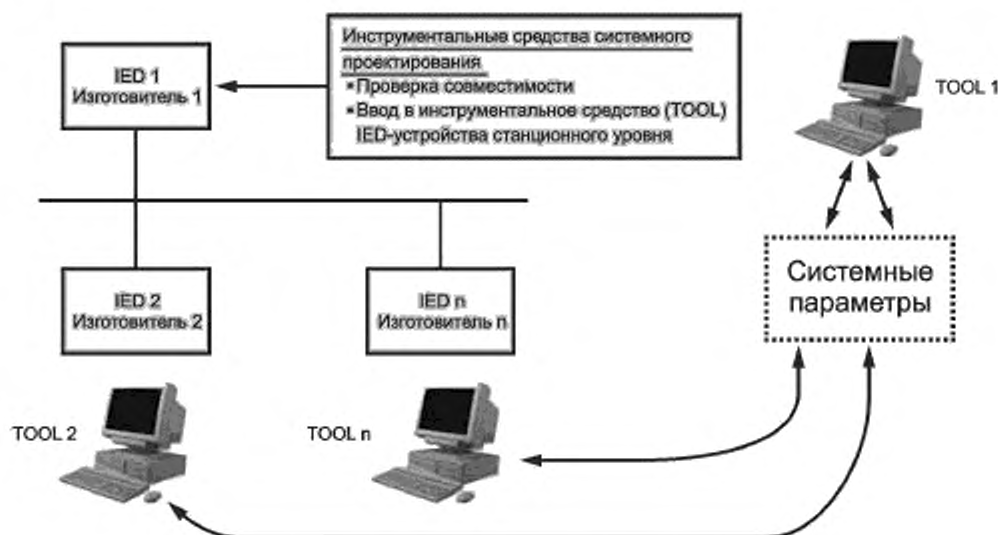
Рисунок 9 — Обмен системными параметрами
