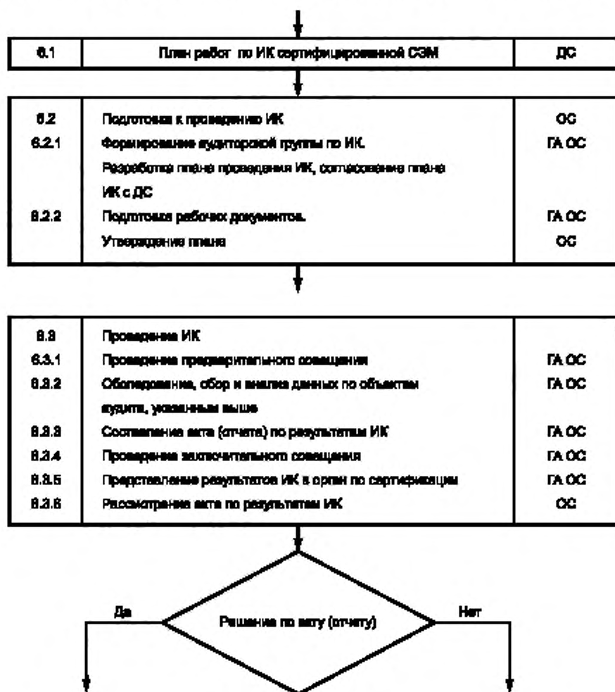
Стадия 6. Последовательность процедур инспекционного контроля сертифицированной СЭМ
