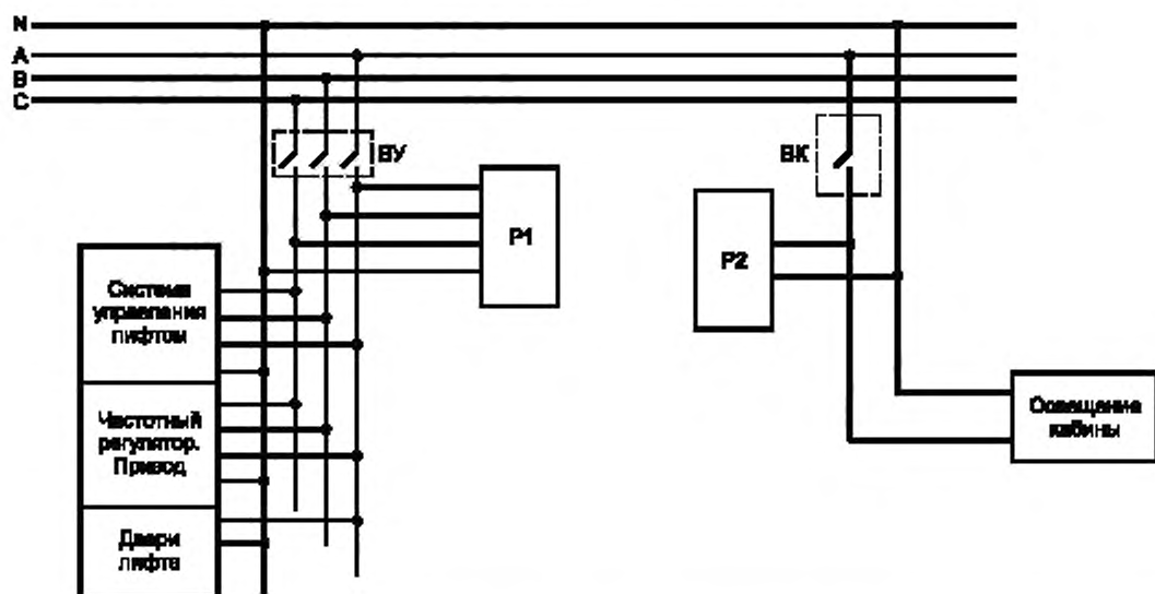
Структурная схема подключения приборов для измерения потребления электроэнергии
