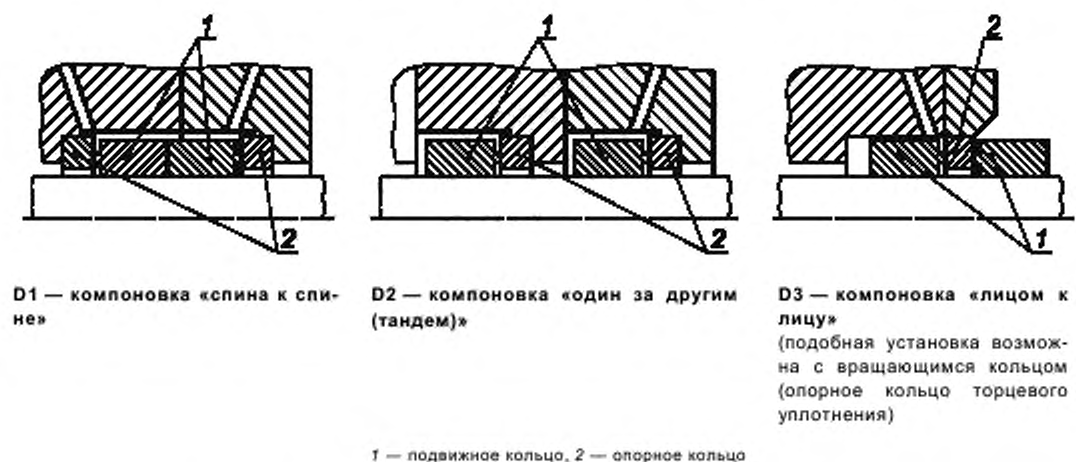
Рисунок D.3 — Примеры компоновок составного торцевого уплотнения
