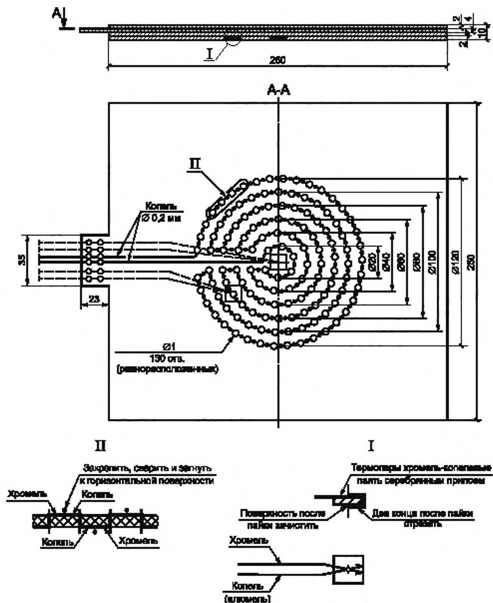
Рисунок 2 — Пример исполнения термомера и закрепленных на нем термодпар
