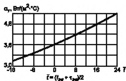
Рисунок Е.2 — График для определения \alpha_r
