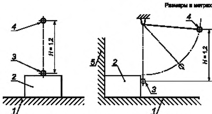
Рисунок 101 — Испытание на удар с применением ударного элемента
