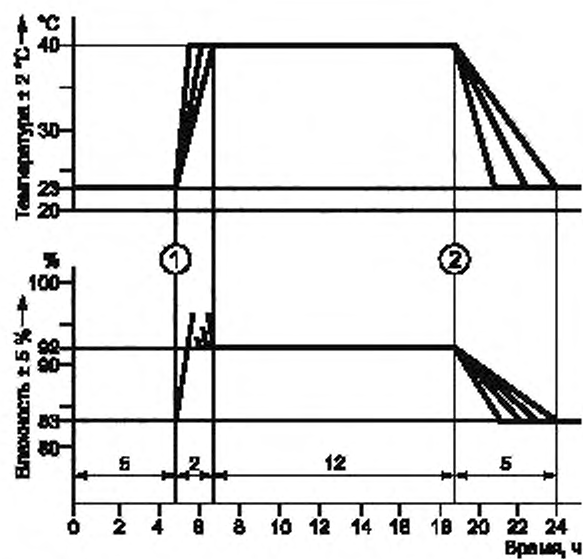
Рисунок 102 — Диаграммы температуры и влажности
