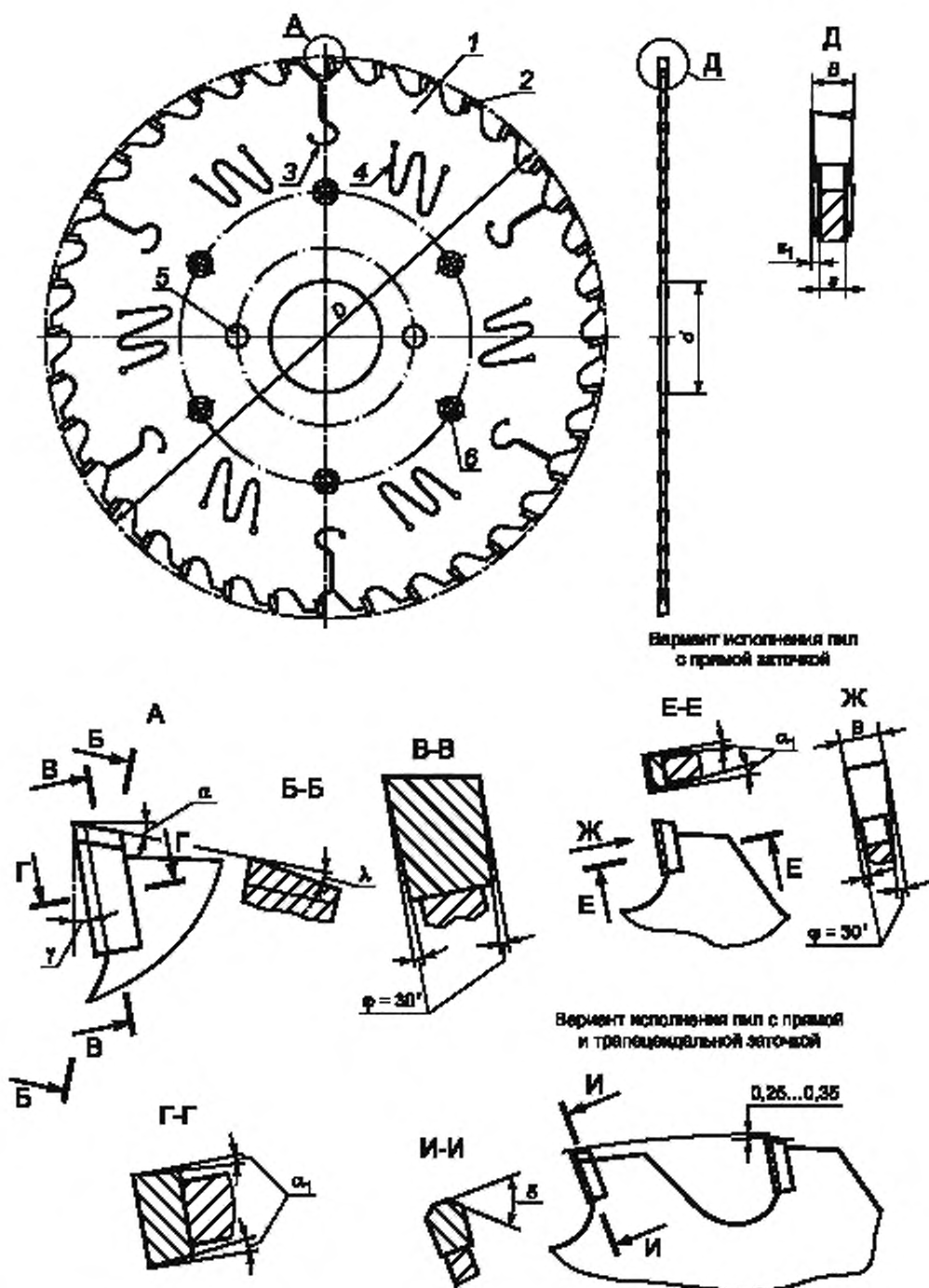
1 — корпус; 2 — пластина из СТМ; 3 — компенсаторы; 4 — отверстия для снижения шума; 5 — отверстия для закрепления и передачи крутящего момента; 6 — отверстия для закрепления пилы на фланце
