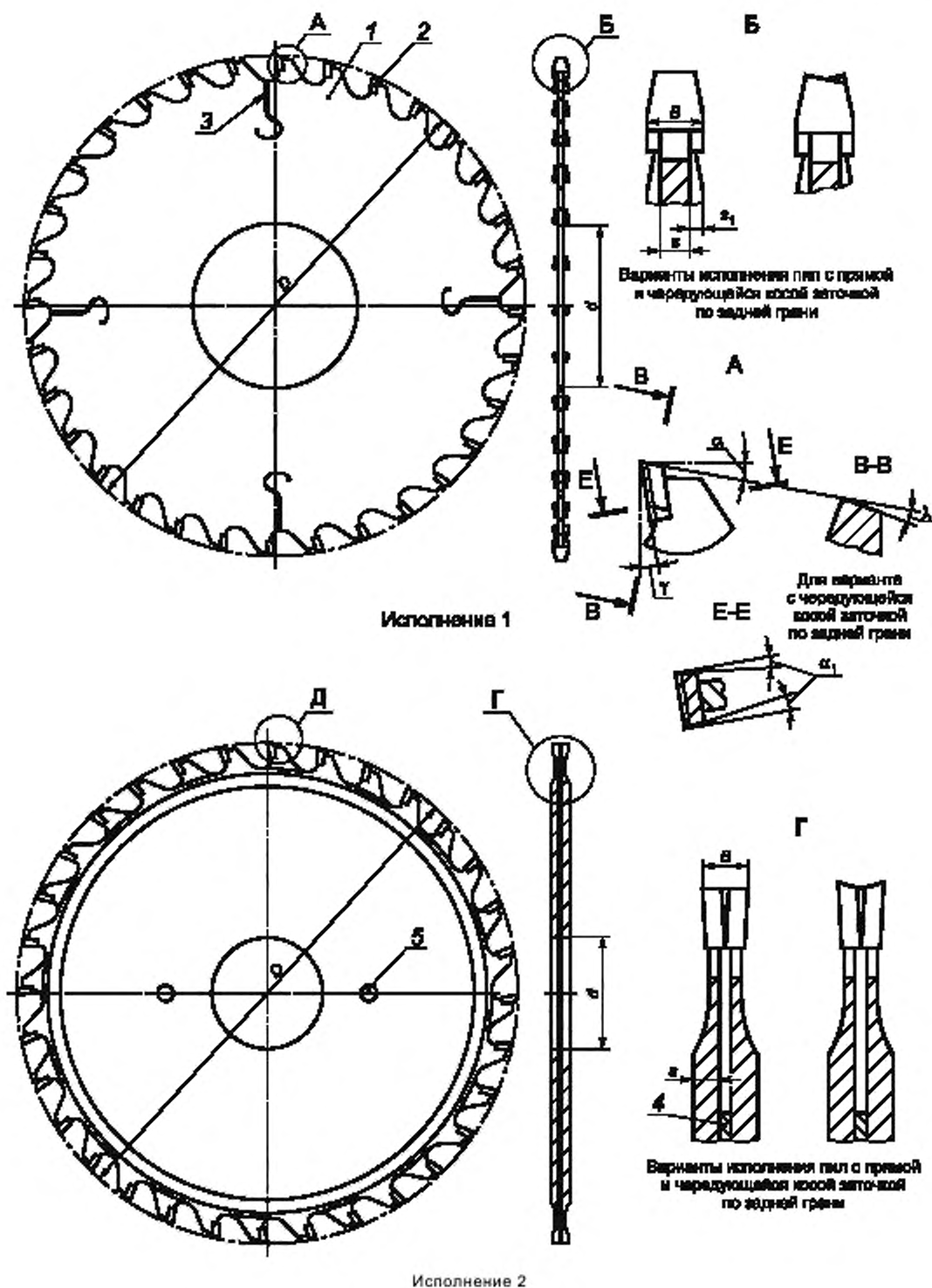
Рисунок 3 — Тип 3, лист 1
