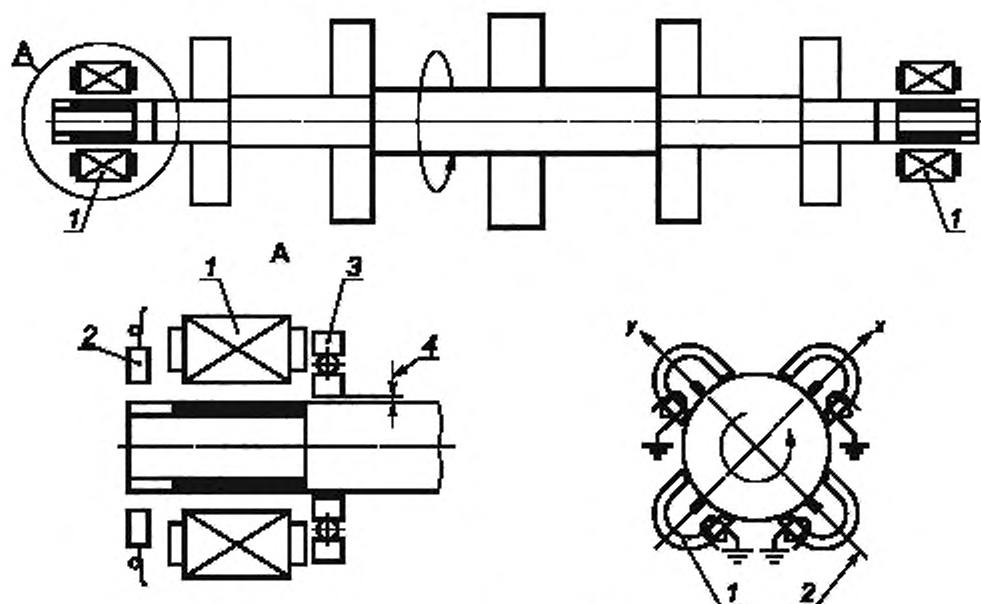
1 — АМП; 2 — датчик перемещения; 3 — страхующий подшипник; 4 — зазор АМП
