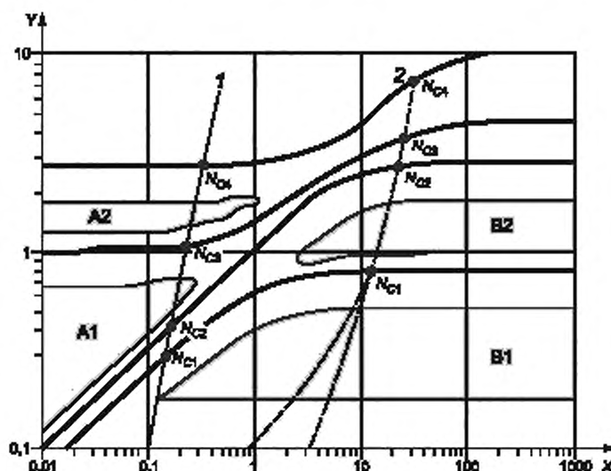
1 — АМП; 2 — подшипник жидкостного трения, X — отношение жесткости подшипника к жесткости вала; Y — отношение частоты собственных колебаний к частоте первой моды собственных изгибных колебания с незакрепленными концами
