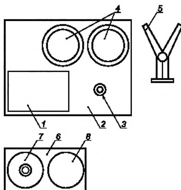
Схема устройства для формовки клейковины
