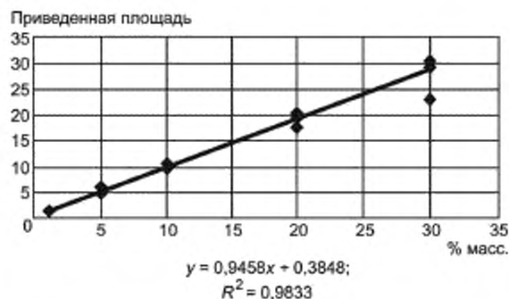
Рисунок А2.4 — Определение расчетного отклика при анализе МТБЗ методом ИНА
