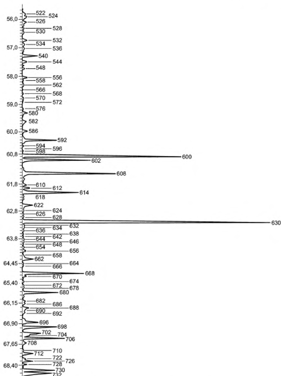
Рисунок X2.10 — Детальная хроматограмма стандартного образца бензина CGSB0496 (55,5 — 68,5 мин)
