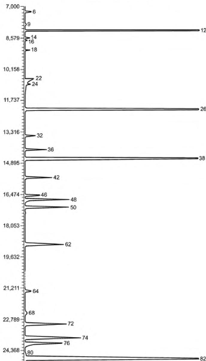
Рисунок 1 — Хроматограмма стандартного образца бензина 2)
