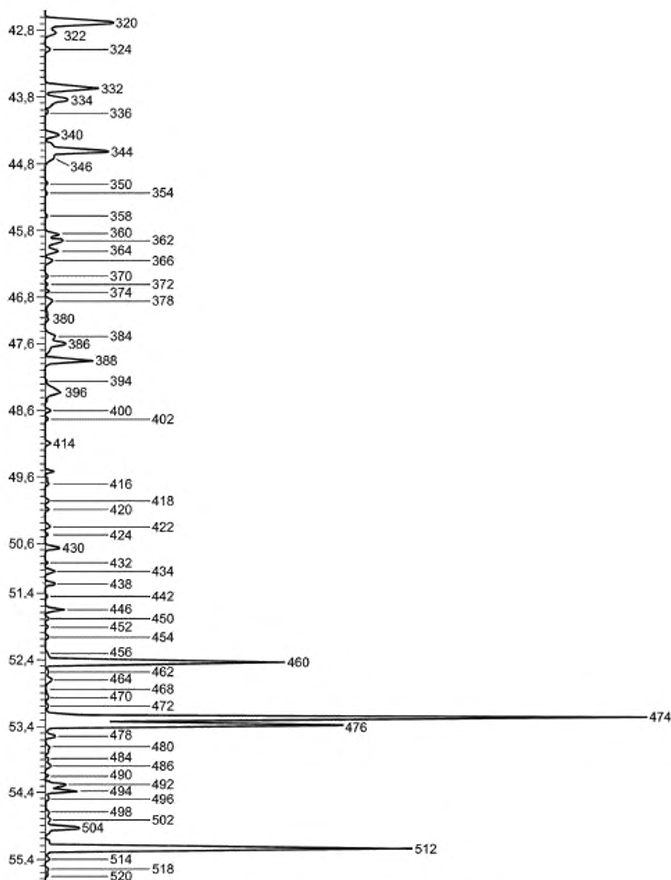
Рисунок X2.9 — Детальная хроматограмма стандартного образца бензина CGSB0496 (42,5 — 55,5 мин)
