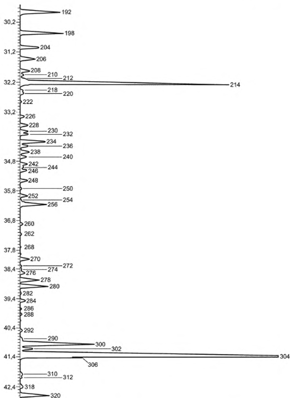
Рисунок X2.8 — Детальная хроматограмма стандартного образца бензина CGSB0496 (30,5 — 42,5 мин)
