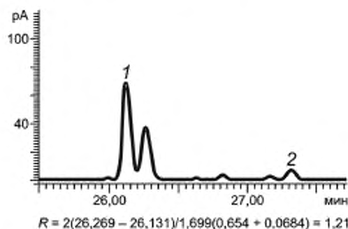
Рисунок X2.2 — Бензол и 1-метилциклопентен
