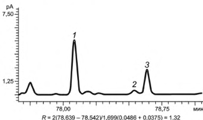
Рисунок X2.5 — Тридекан и 1-метилнафталин
