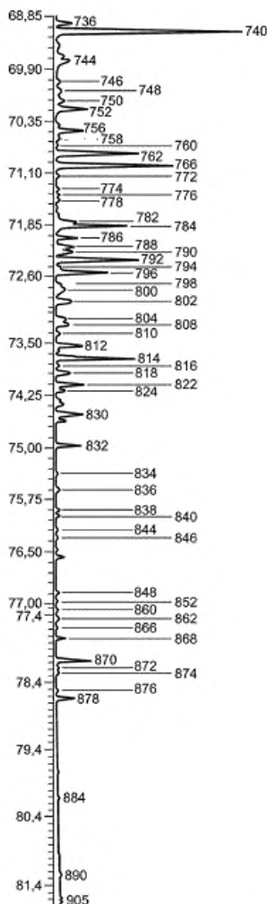
Рисунок X2.11 — Детальная хроматограмма стандартного образца бензина CGSB0496 (68,5 — 82 мин)
