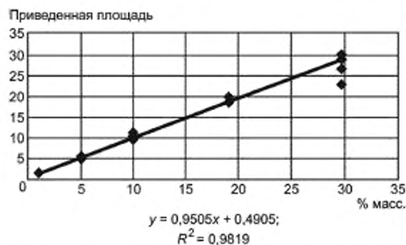
Рисунок А2.6 — Определение расчетного отклика при анализе ТАМЗ методом ИНА
