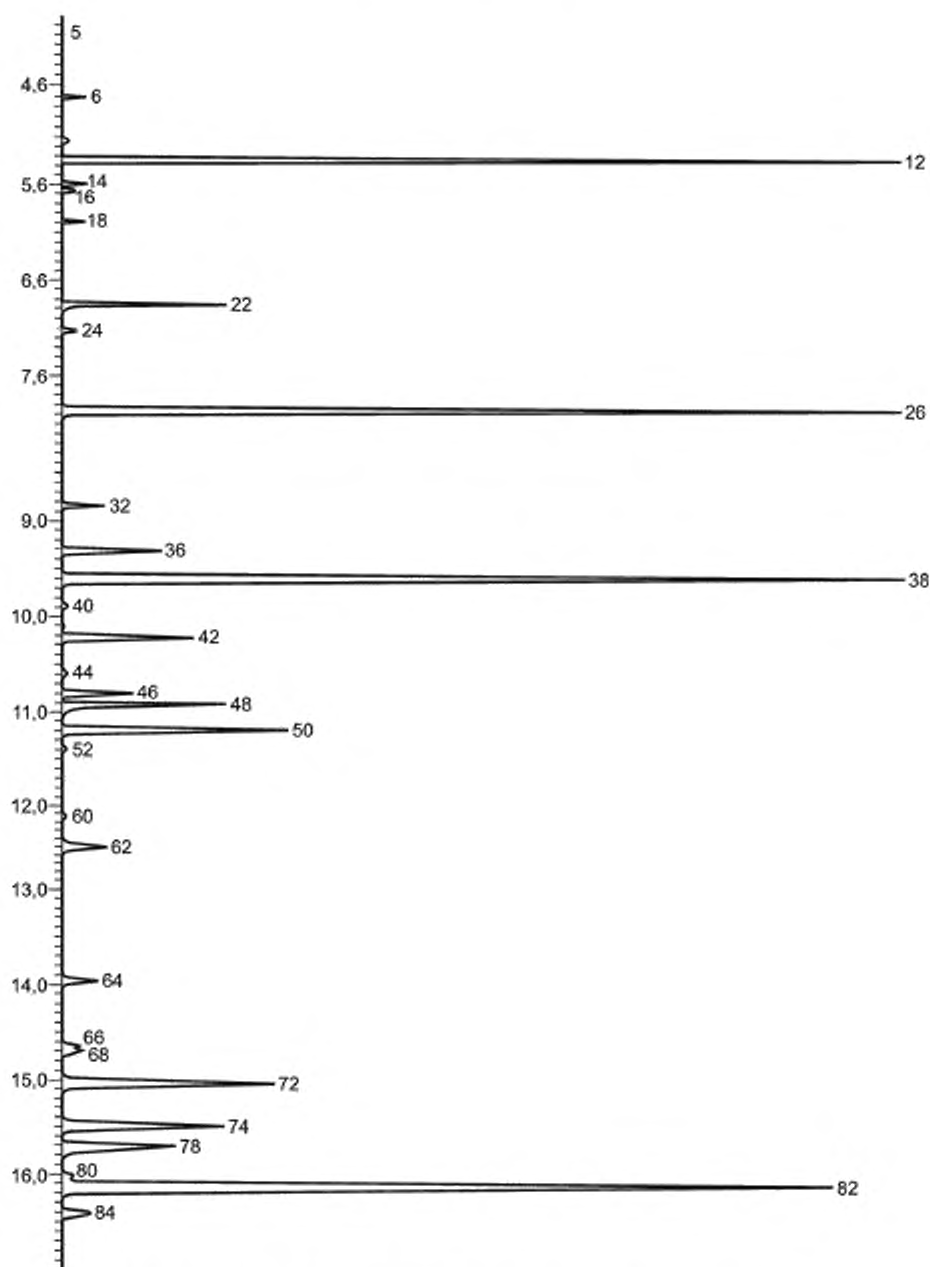
Рисунок X2.6 — Детальная хроматограмма стандартного образца бензина CGSB0496 (0 — 17 мин)
