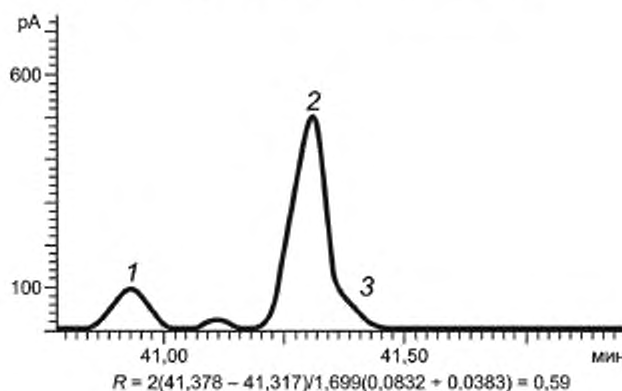
Рисунок X2.2 — Бензол и 1-метилциклопентен
