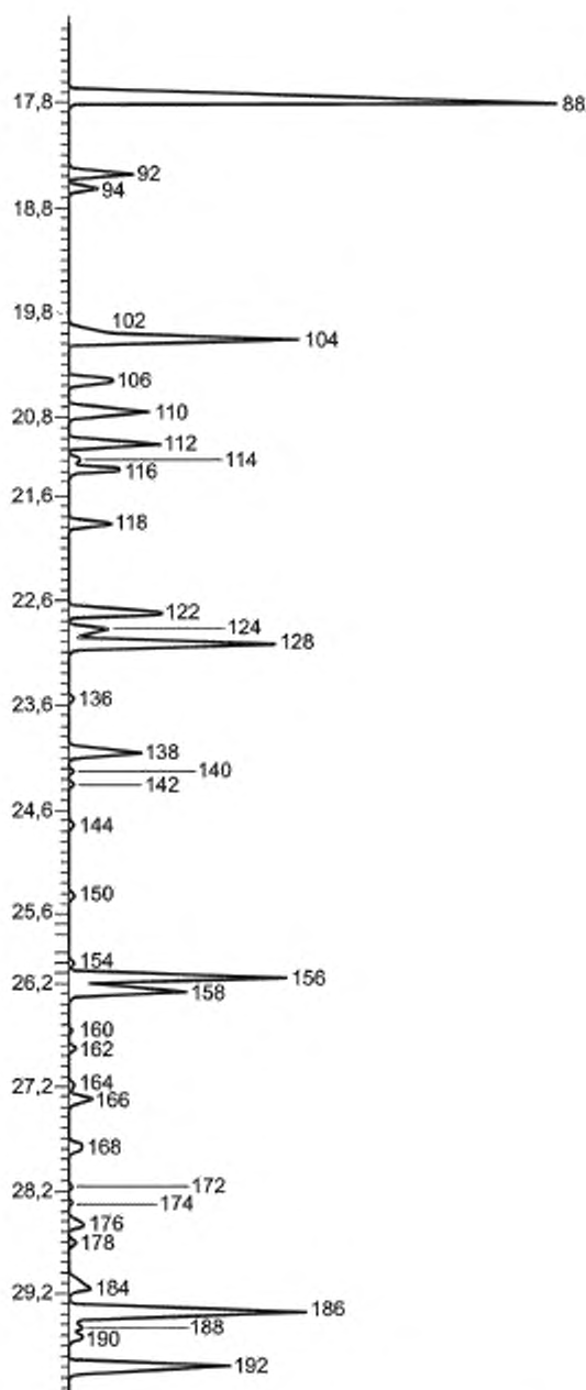
Рисунок X2.7 — Детальная хроматограмма стандартного образца бензина CGSB0496 (17 — 30,5 мин)
