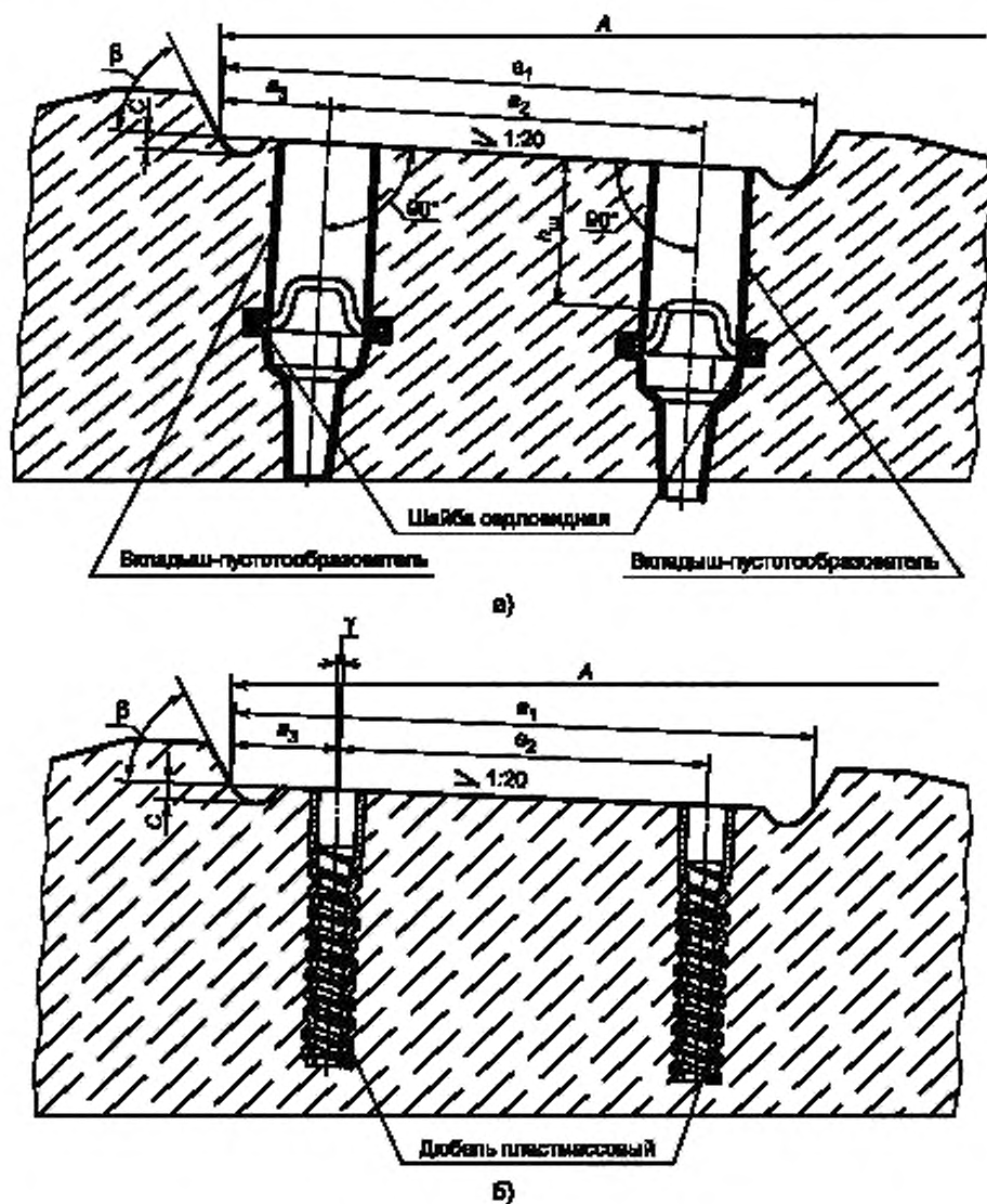
Рисунок 6 — Подрельсовая часть шпал типа III
