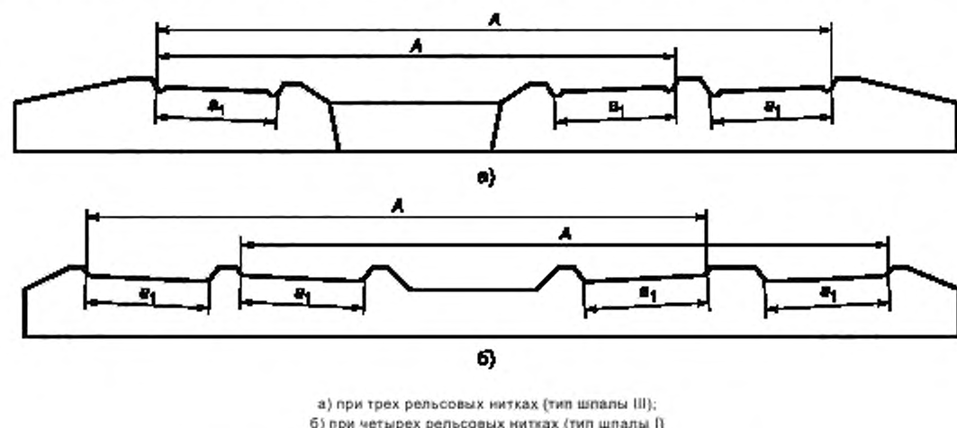
Рисунок 4 — Схема шпал с совмещенной колеей разной ширины
