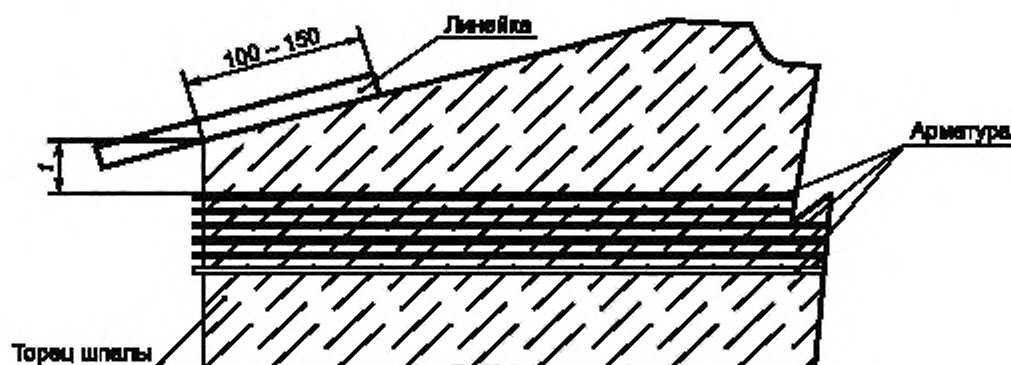
Рисунок 21 — Схема определения толщины t защитного слоя бетона
