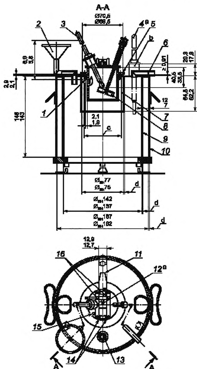
1 — эбонитовое или фибровое кольцо (удобная, легкая подгонка на тигле); 2 — воронка; 3 — термометр для тигля; 4 — термометр для обогревающего сосуда; 5 — 2,2 \times 3,8 для длинных винтов CSK; 6 — медная переливная трубка; 7 — внутренняя (воздушная) камера; 8 — мешалка; 9 — сосуд для обогрева; 10 — наружный кожух; 11 — задвижка, латунь 20 SWG 0,91; 12 — газовая форсунка или сигнальная лампочка; 13 — термометр для обогревающего сосуда; 14 — направляющие; 15 — белая бусинка из пригодного материала диаметром 3,6—4,1 мм; 16 — кольца цапф; а — вид сверху относительно действительного положения; б — внутренний диаметр гнезда термометра 15—15,5 мм; с — зазор в верхней пластине 2,5 мм, не более; д — медь 0,6; е — длина жиклера приблизительно 15 мм; отверстие на конце жиклера не более 1,71 и не менее 1,48 мм
