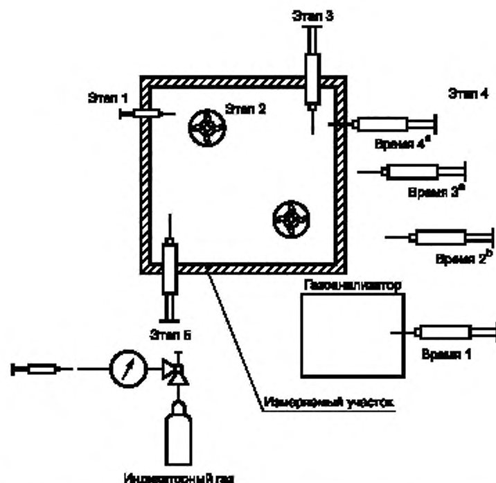
Рисунок 1 — Общая схема метода установки и этапов снижения концентрации индикаторного газа
