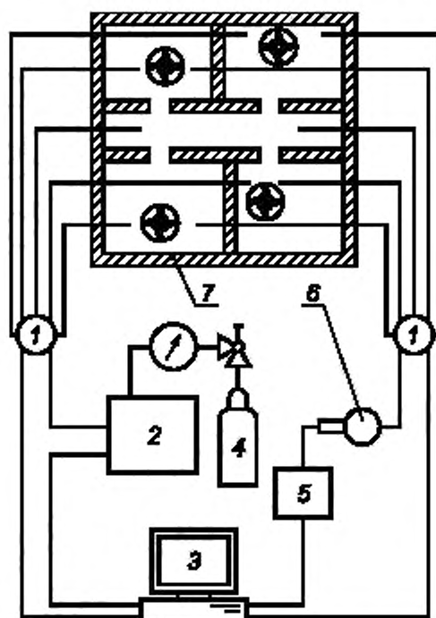
1 — коллектор; 2 — газ; 3 — обработка данных; 4 — индикаторный газ; 5 — газоанализатор; 6 — насос; 7 — исследуемый участок
