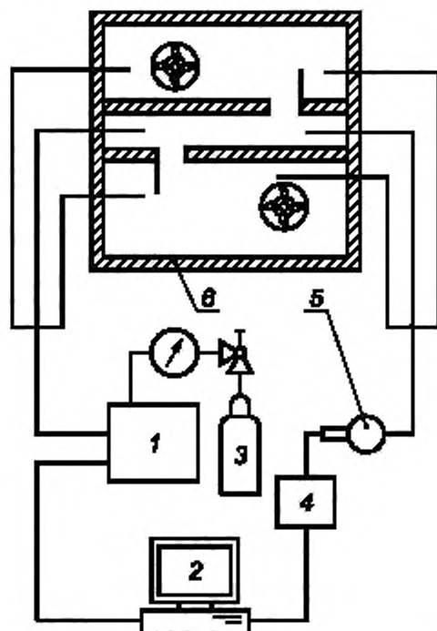
1 — газ; 2 — обработка данных; 3 — индикаторный газ; 4 — газоанализатор; 5 — насос; 6 — исследуемый участок
