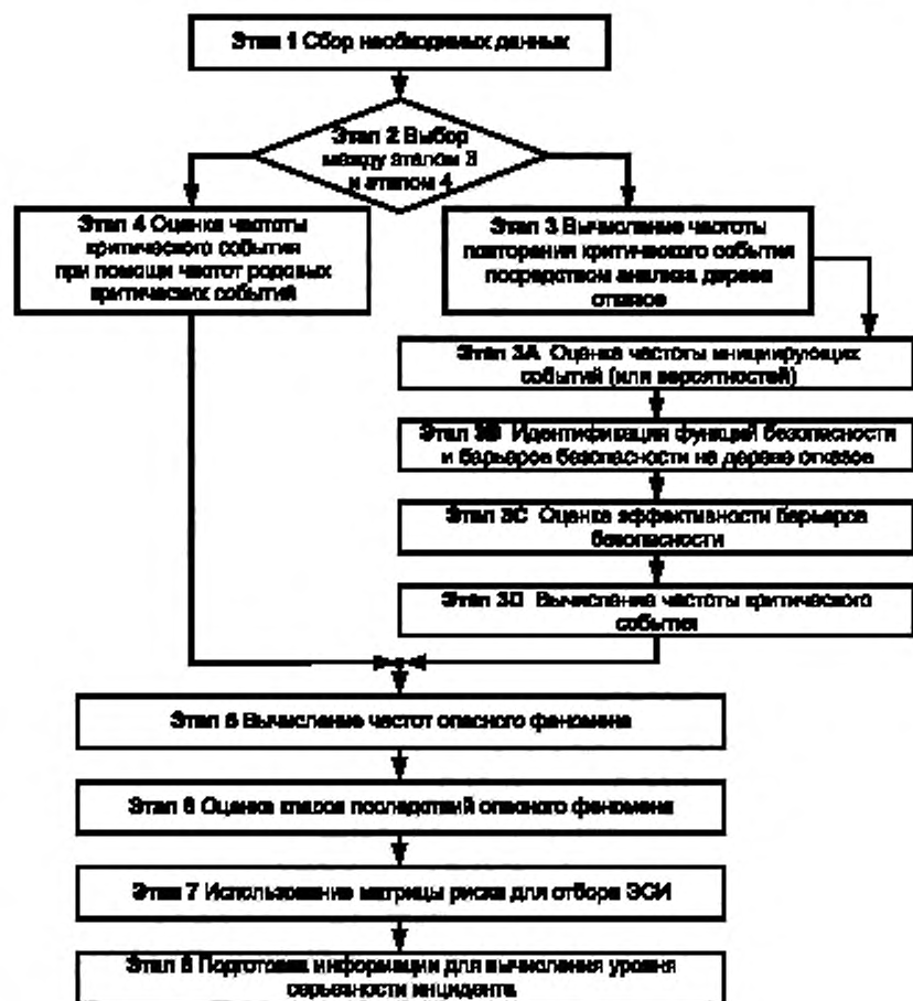
Рисунок 1 — Общая схема этапов МИЗСИ
