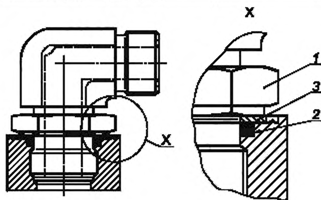
1 — установочная гайка; 2 — О-образное уплотнительное кольцо; 3 — защитная (фиксирующая) шайба
